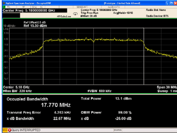
802.11n(HT20) U-NII-1 Low CH
