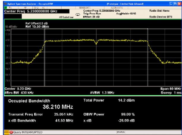
802.11 n(HT40) U-NII-1 High CH
