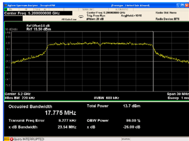
802.11a U-NII-1 Middle CH
