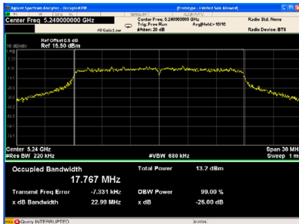
802.11 ac(HT20) U-NII-1 High CH
