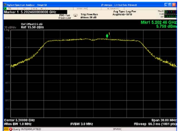
802.11ac(HT20) U-NII-1 Middle CH
