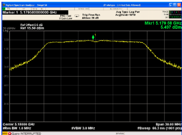
802.11ac(HT20) U-NII-1 Low CH
