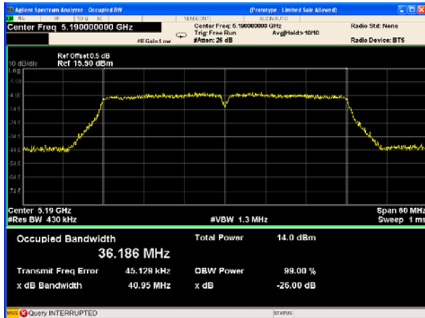
802.11n(HT40) U-NII-1 Low CH
