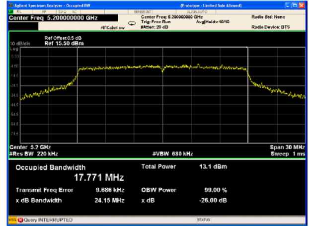
802.11 n(HT20) U-NII-1 Middle CH
