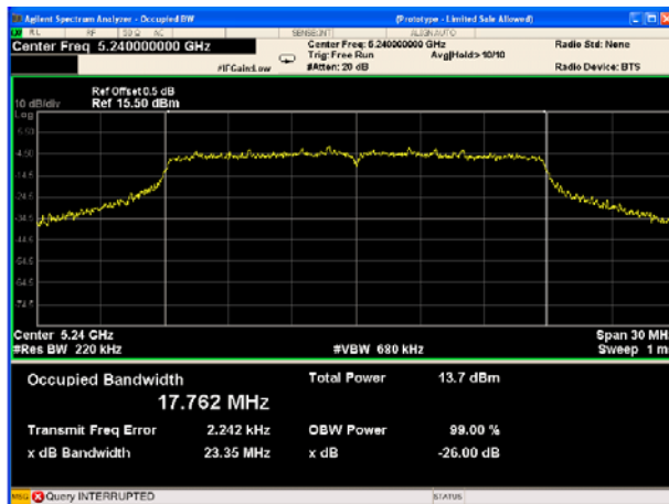
802.11n(HT20) U-NII-1 High CH
