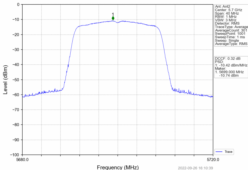
802.11n(HT20)_HCH_5700MHz_Ant2_NTNV
