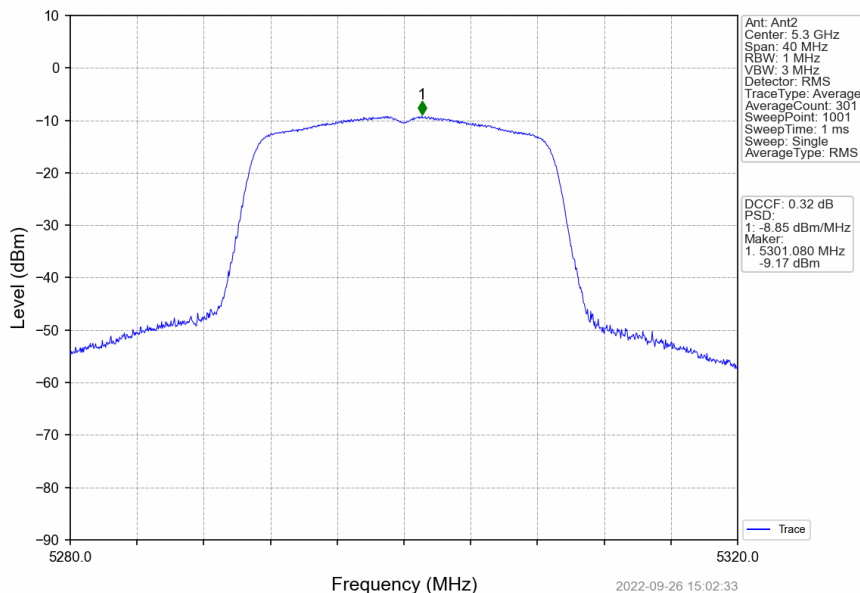
802.11n(HT20)_MCH_5300MHz_Ant2_NTNV
