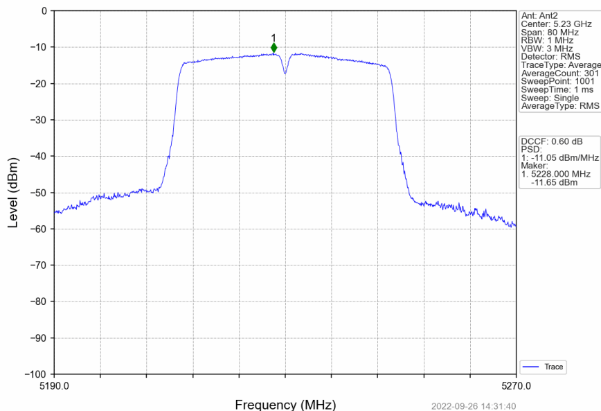
802.11n(HT40)_HCH_5230MHz_Ant2_NTNV
