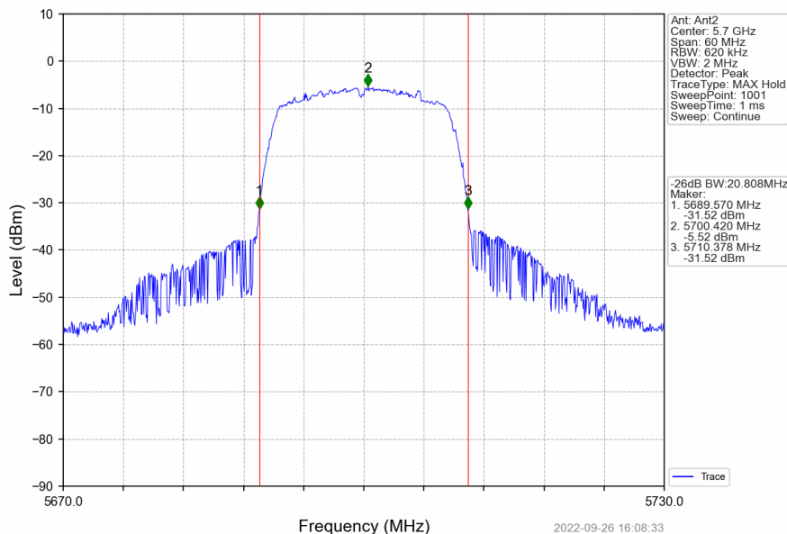
802.11n(HT20)_HCH_5700MHz_Ant2_NTNV
