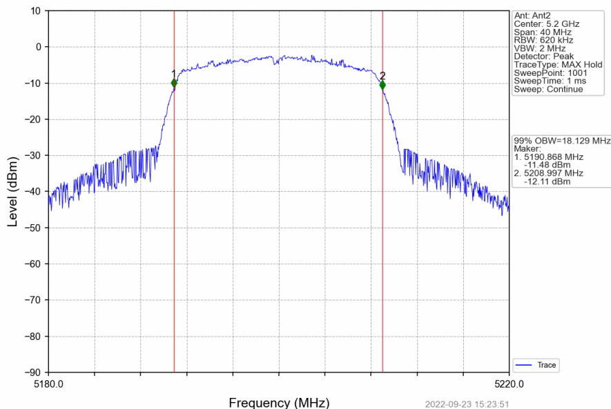
802.11n(HT20)_MCH_5200MHz_Ant2_NTNV
