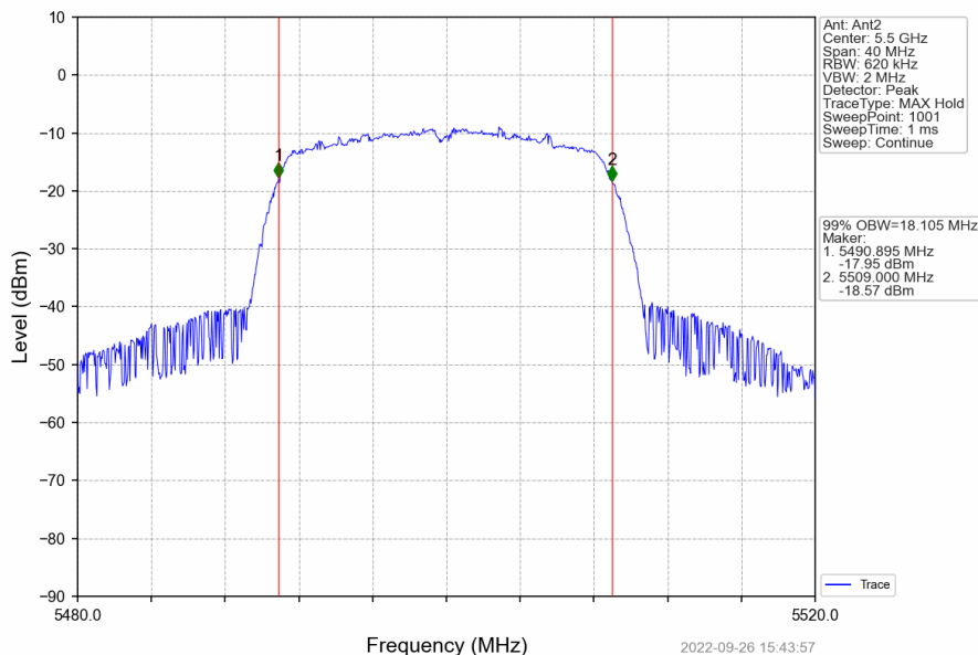
802.11n(HT20)_LCH_5500MHz_Ant2_NTNV
