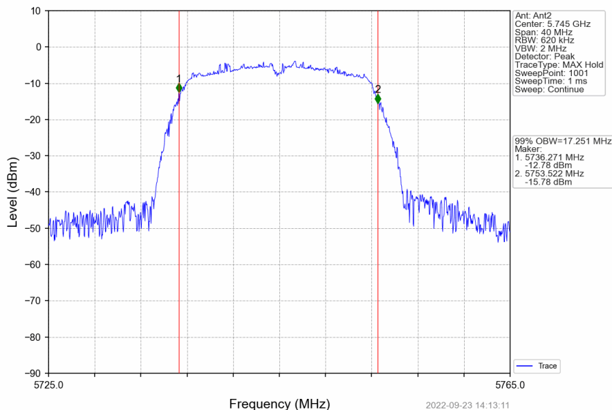
802.11a_LCH_5745MHz_Ant2_NTNV
