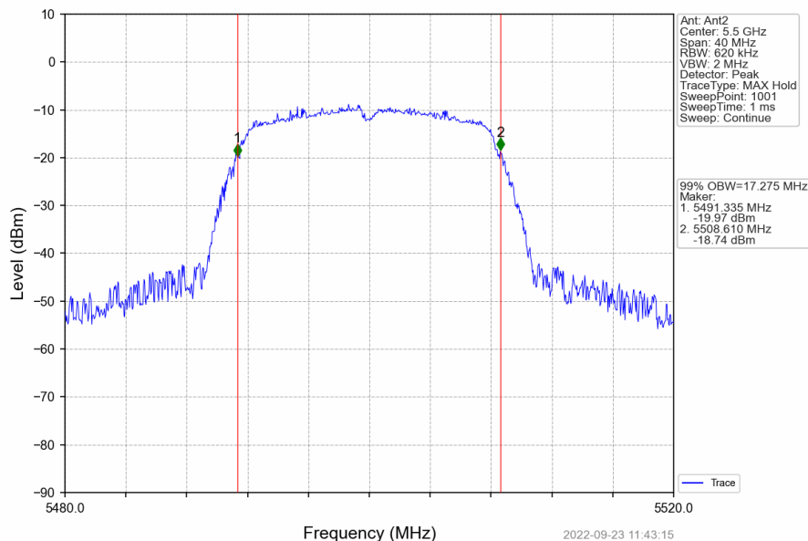
802.11a_LCH_5500MHz_Ant2_NTNV
