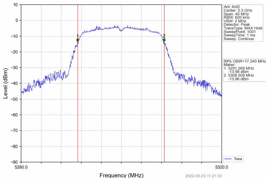
802.11a_MCH_5300MHz_Ant2_NTNV
