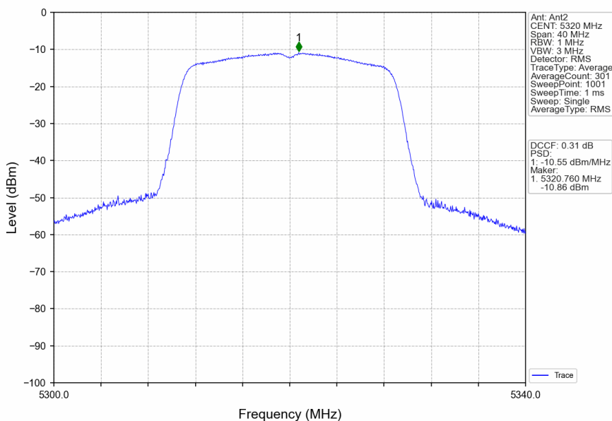
802.11n(HT20)_HCH_5320MHz_MIMO_NTNV
