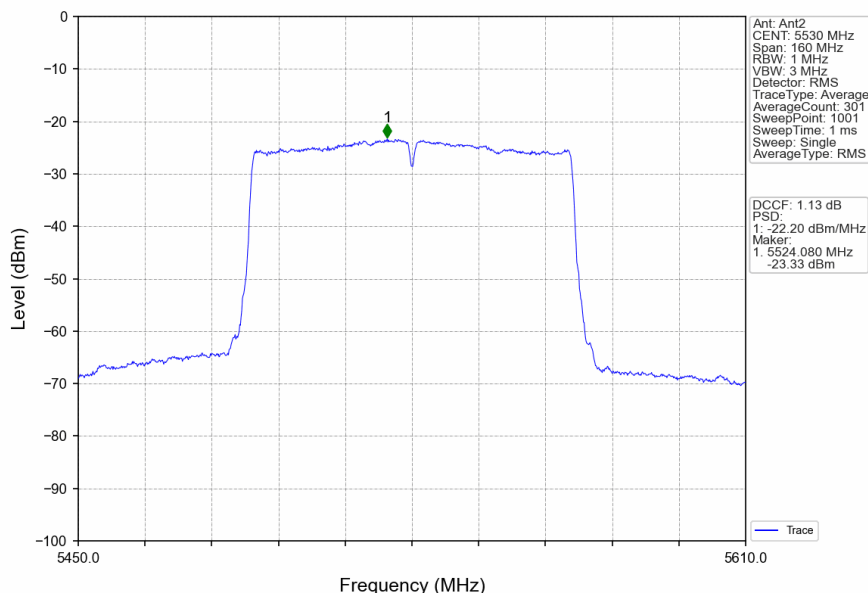
802.11ac(VHT80)_LCH_5530MHz_Ant2_NTNV
