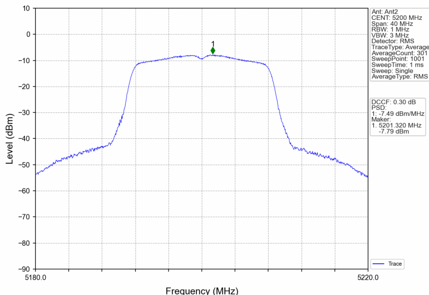
802.11a_MCH_5200MHz_Ant2_NTNV
