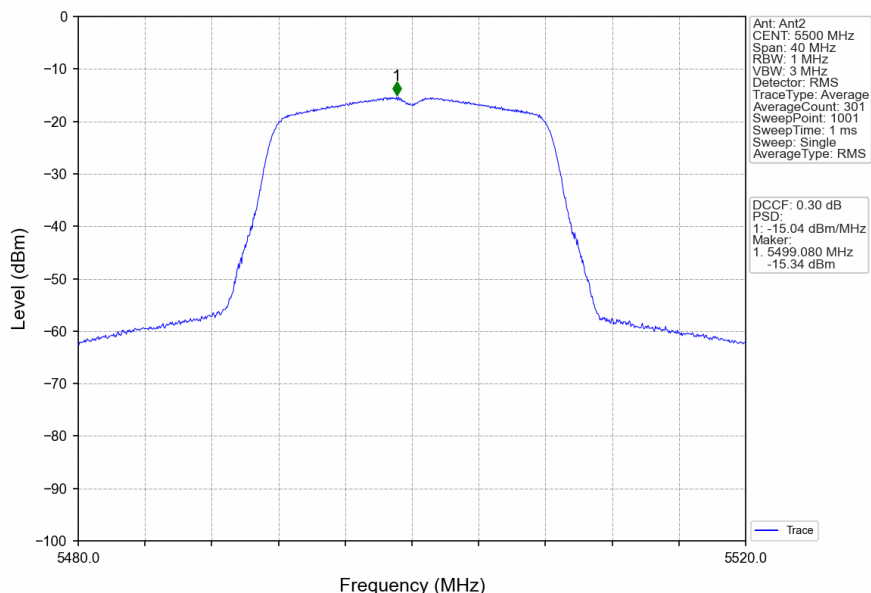
802.11a_LCH_5500MHz_Ant2_NTNV
