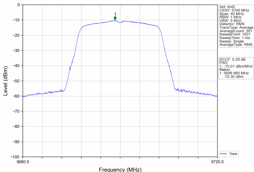
802.11a_HCH_5700MHz_Ant2_NTNV
