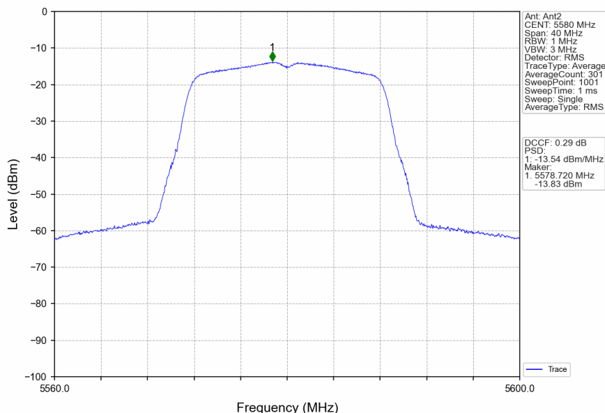
802.11a_MCH_5580MHz_Ant2_NTNV
