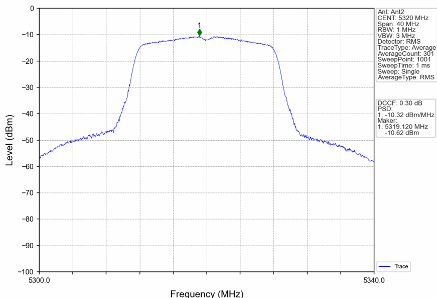
802.11a_HCH_5320MHz_Ant2_NTNV
