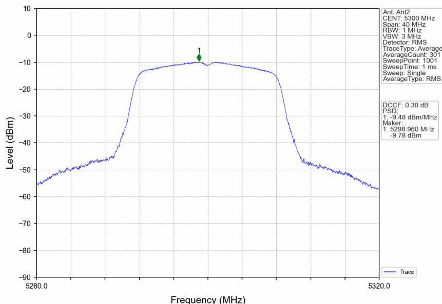
802.11a_MCH_5300MHz_Ant2_NTNV
