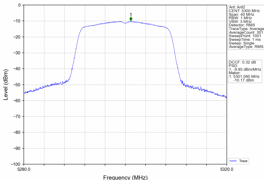
802.11n(HT20)_MCH_5300MHz_Ant2_NTNV
