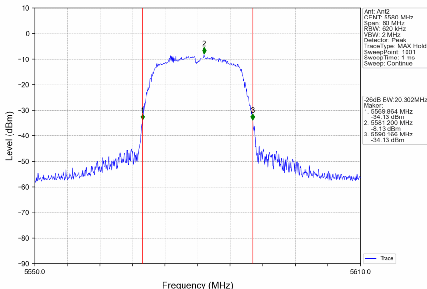
802.11a_MCH_5580MHz_Ant2_NTNV
