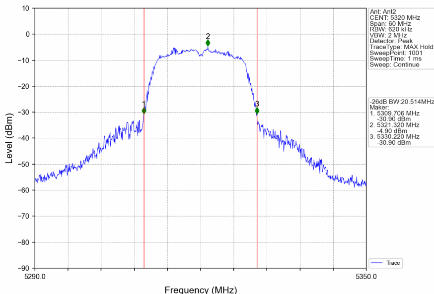
802.11a_HCH_5320MHz_Ant2_NTNV
