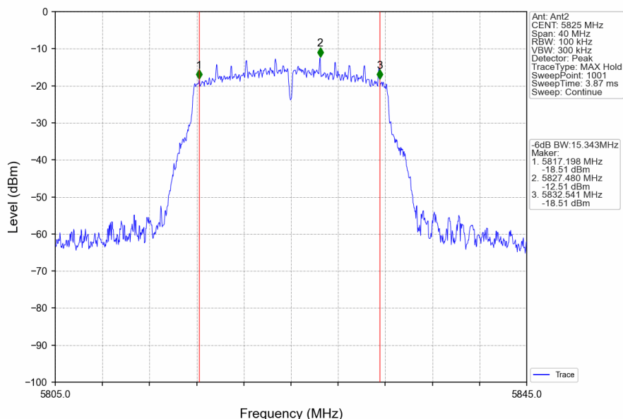
802.11a_HCH_5825MHz_Ant2_NTNV
