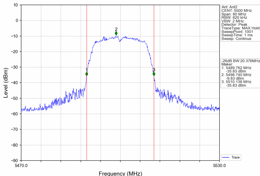
802.11a_LCH_5500MHz_Ant2_NTNV
