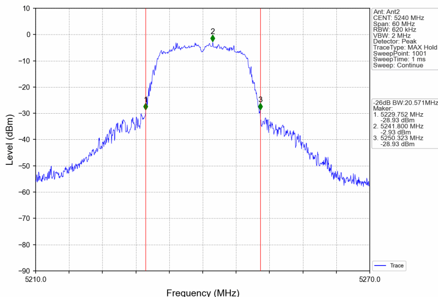
802.11a_HCH_5240MHz_Ant2_NTNV
