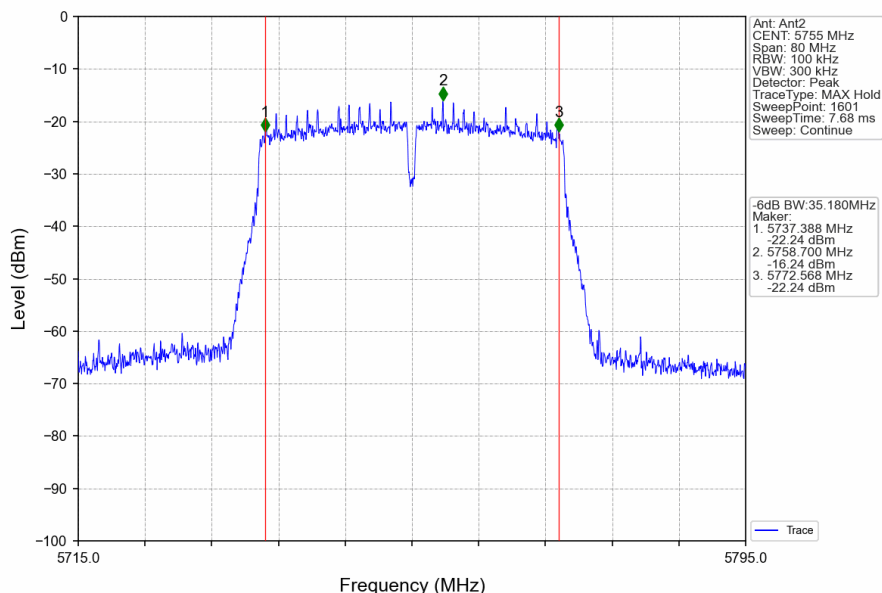
802.11ac(VHT40)_LCH_5755MHz_Ant2_NTNV
