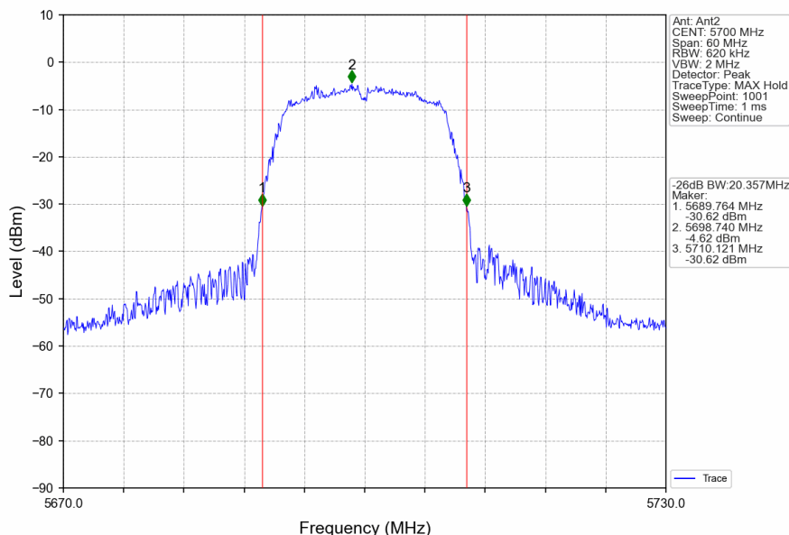
802.11a_HCH_5700MHz_Ant2_NTNV
