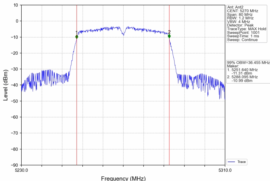
802.11n(HT40)_LCH_5270MHz_Ant2_NTNV
