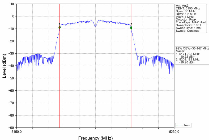
802.11n(HT40)_LCH_5190MHz_Ant2_NTNV
