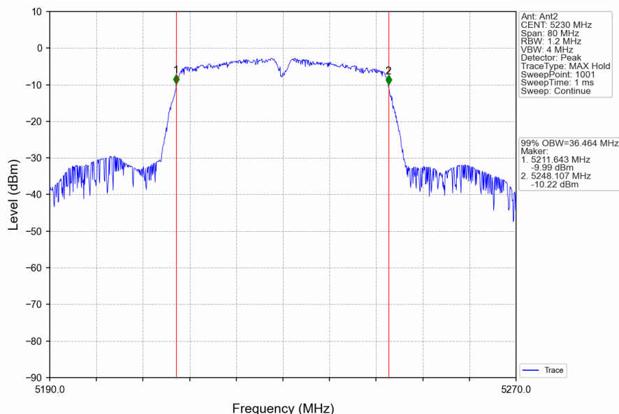
802.11n(HT40)_HCH_5230MHz_Ant2_NTNV
