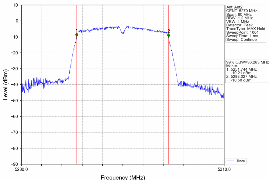
802.11ac(VHT40)_LCH_5270MHz_Ant2_NTNV
