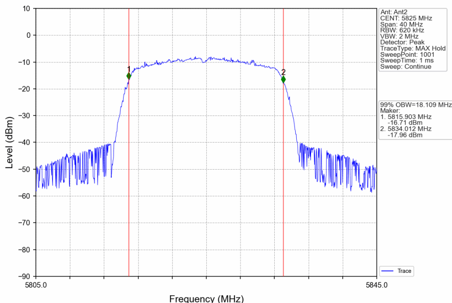
802.11n(HT20)_HCH_5825MHz_Ant2_NTNV
