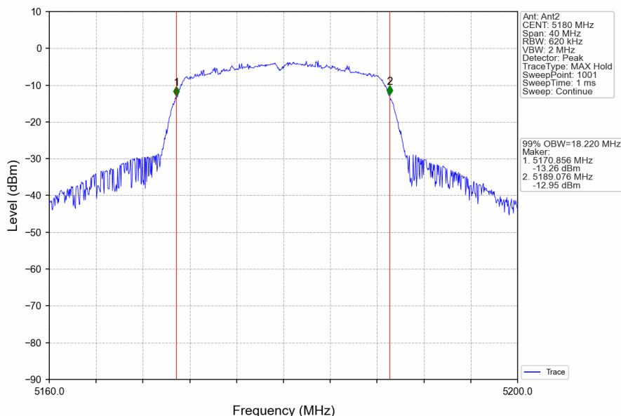
802.11n(HT20)_LCH_5180MHz_Ant2_NTNV
