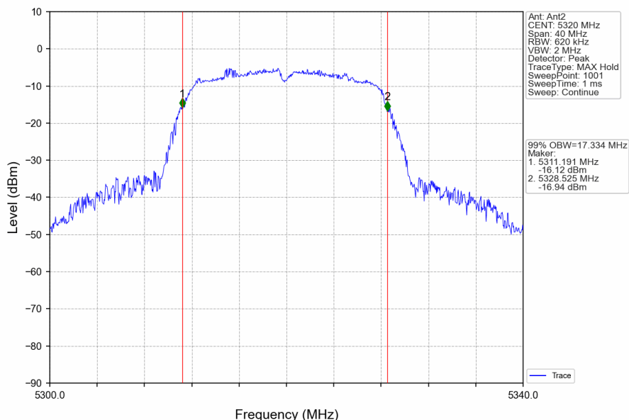
802.11a_HCH_5320MHz_Ant2_NTNV
