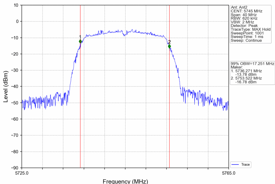
802.11a_LCH_5745MHz_Ant2_NTNV
