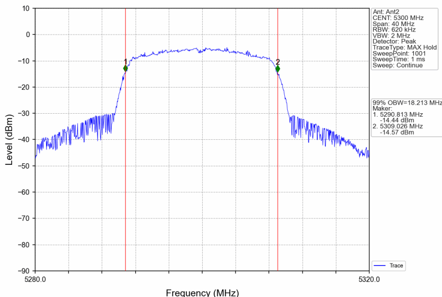
802.11n(HT20)_MCH_5300MHz_Ant2_NTNV
