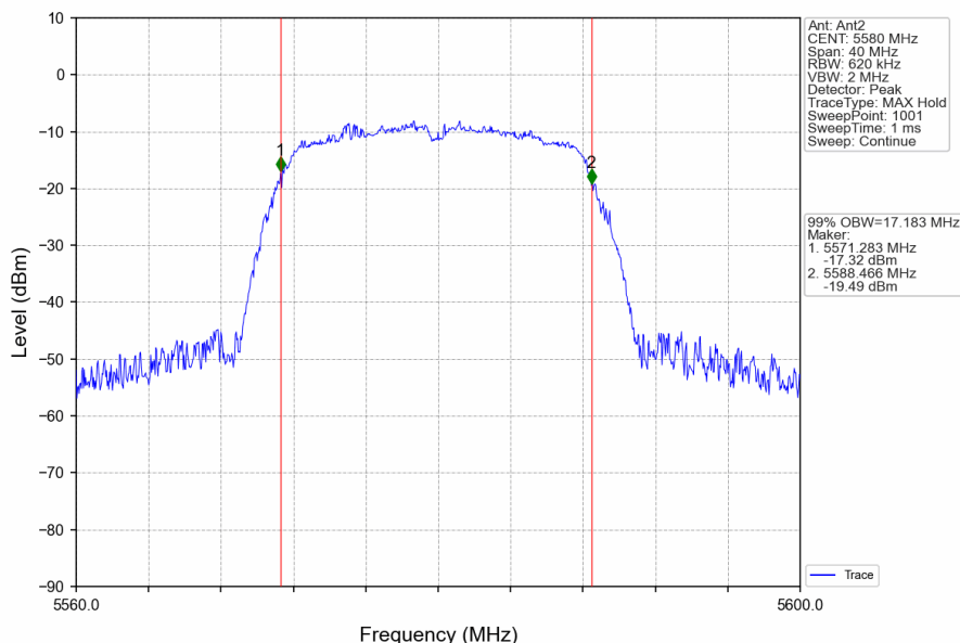
802.11a_MCH_5580MHz_Ant2_NTNV
