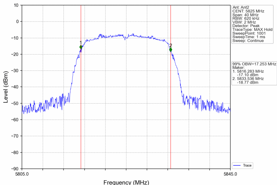
802.11a_HCH_5825MHz_Ant2_NTNV
