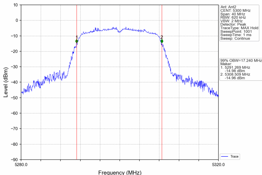
802.11a_MCH_5300MHz_Ant2_NTNV
