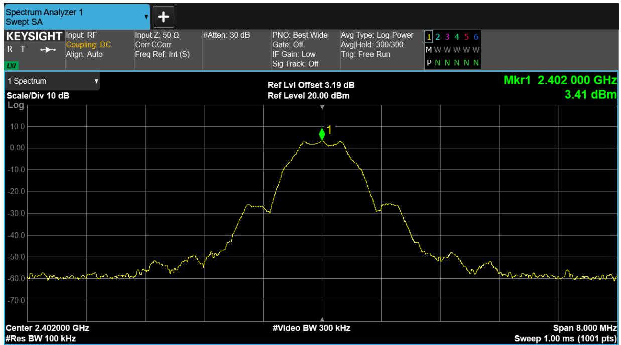
Band Edge NVNT BLE 2402MHz Ant1 Emission
