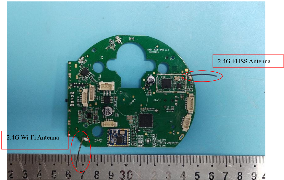
Antenna
