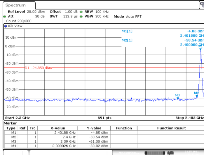
DH5_Ant1_Low_2402
