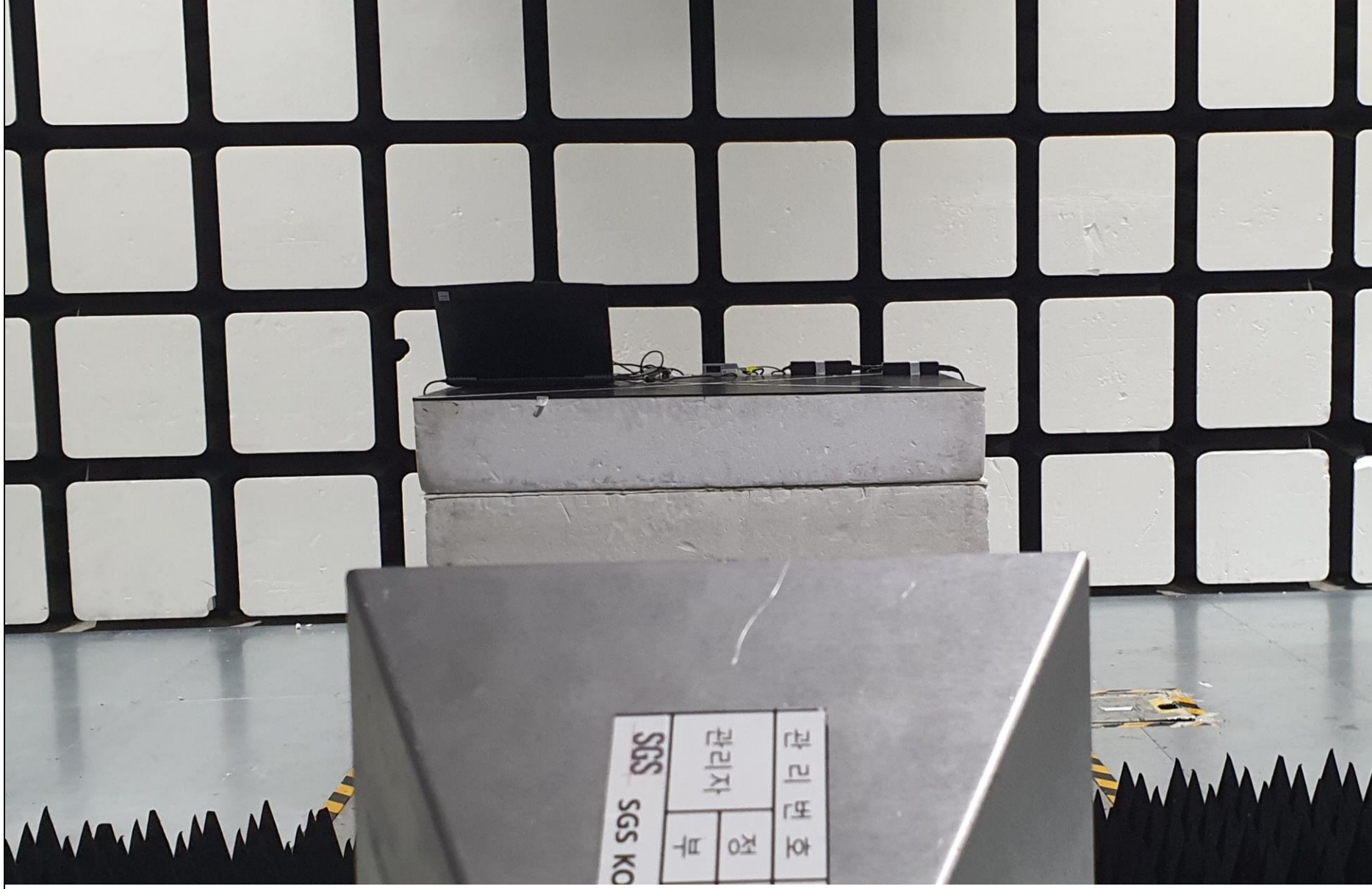
RE(Above 1 GHz)_Front
