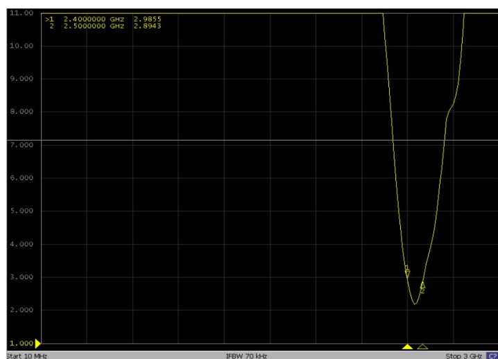
VSWR
