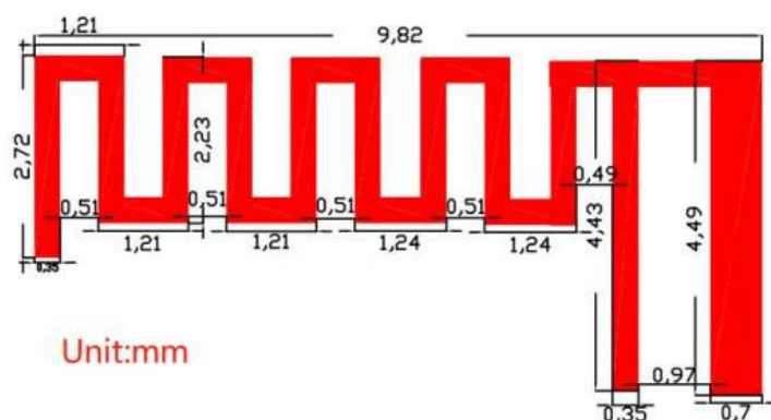
图1- 1 : WLT8016模块
