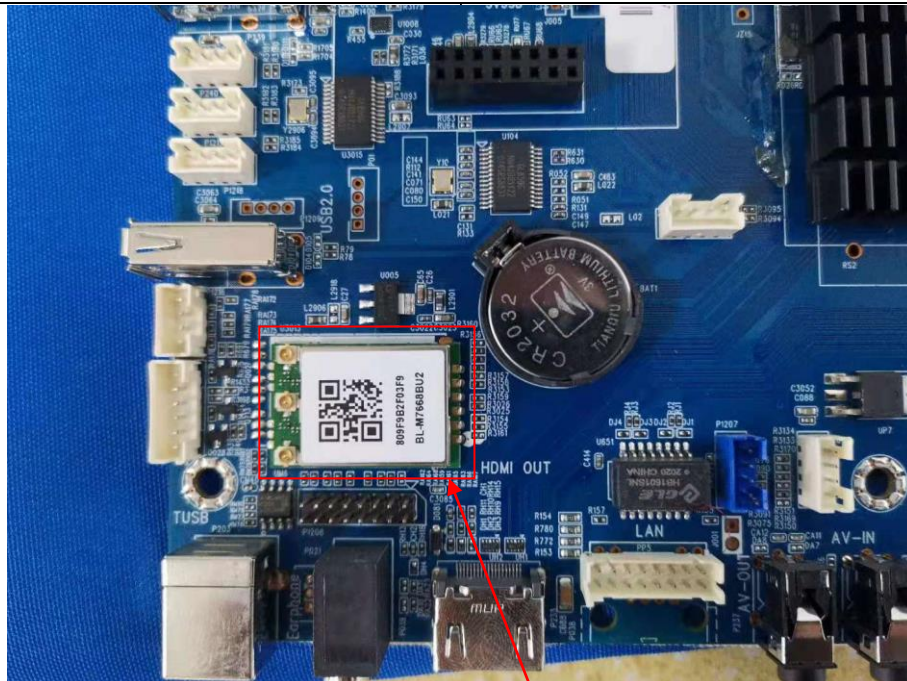
Module BL-M7668BU2
