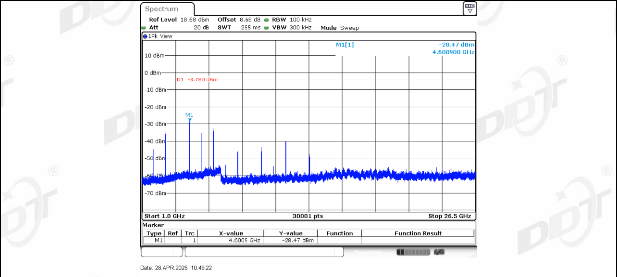
SRD_Ant1_920_1000~26500
