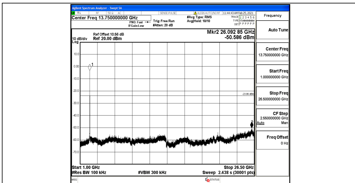
11N20MIMO_Ant2_2437_0-Reference
