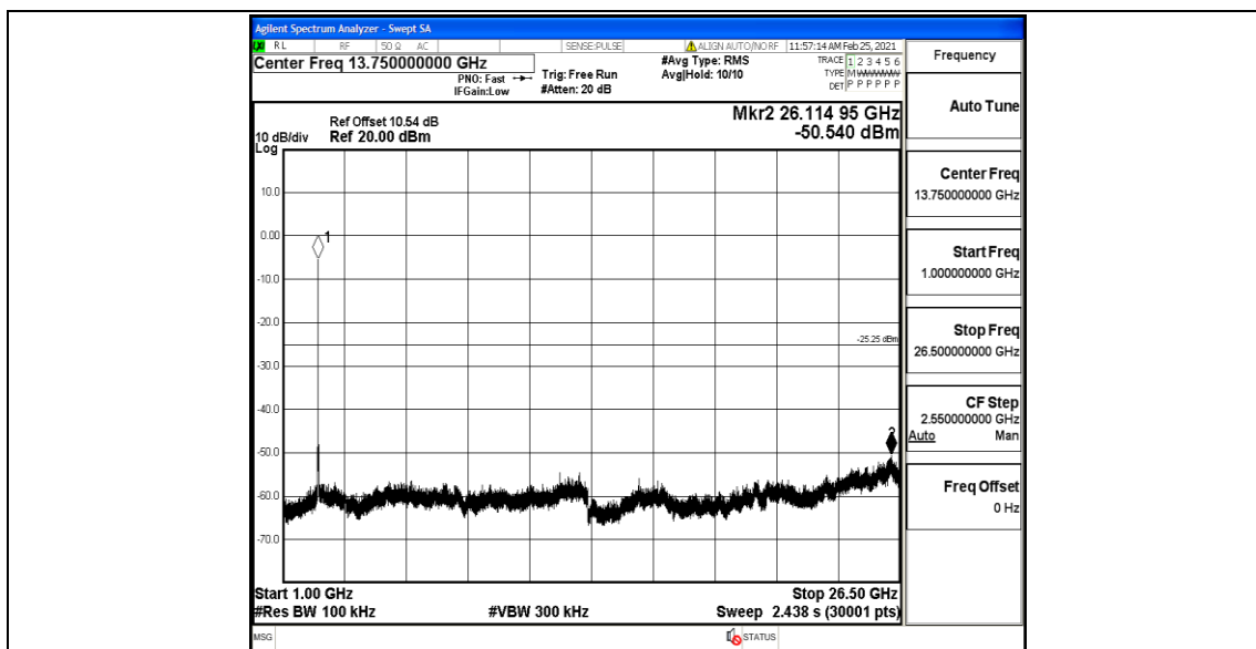
11N40MIMO_Ant1_2422_0~Reference
