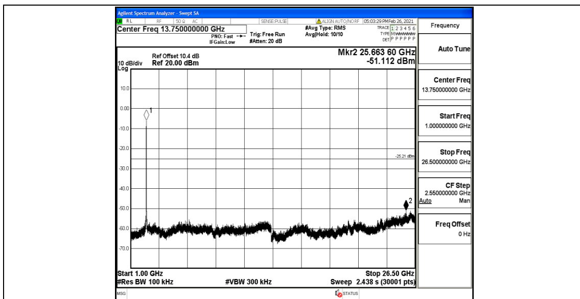
11N40MIMO_Ant2_2422_0~Reference
