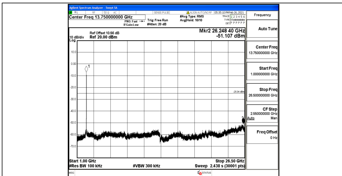
11N40MIMO_Ant2_2437_0-Reference
