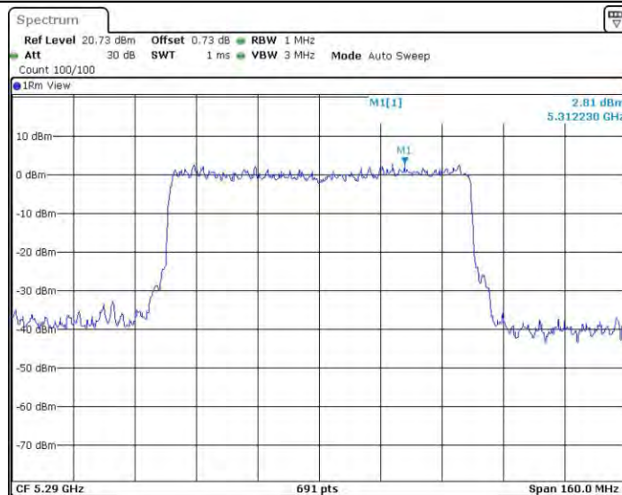
11AX80MIMO_Ant0_5290
