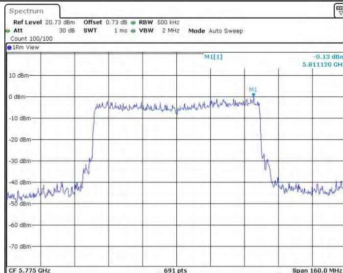
11AX80MIMO_Ant0_5775
