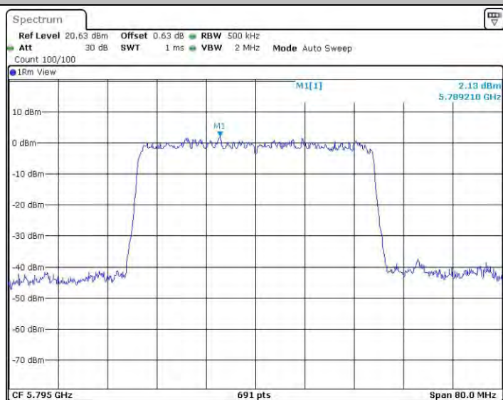
11AX40MIMO_Ant0_5795
