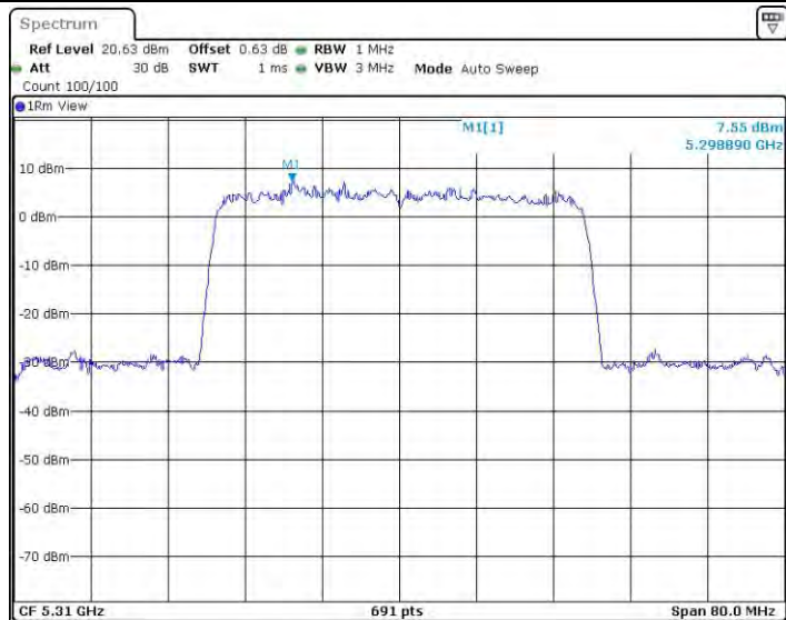
11AX40MIMO_Ant0_5310
