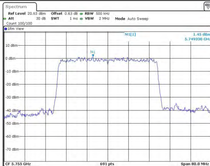
11AX40MIMO_Ant0_5755
