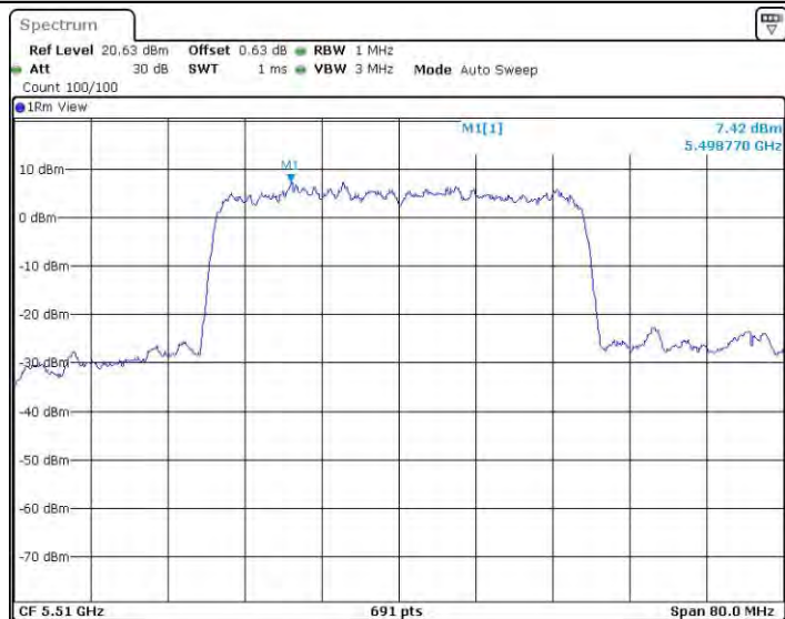
11AX40MIMO_Ant0_5510
