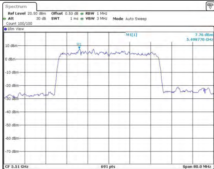
11AX40SISO_Ant0_5510
