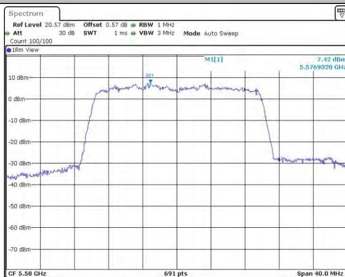
11AX20MIMO_Ant0_5580
