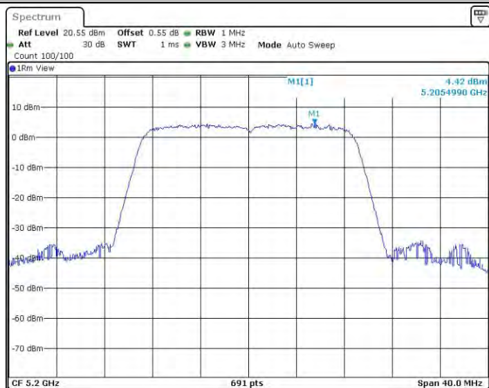
11AC20MIMO_Ant0_5200
