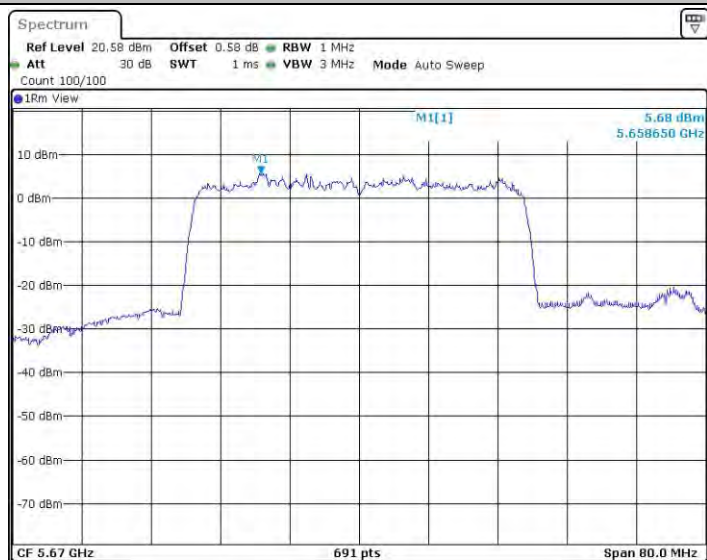
11AX40SISO_Ant0_5670
