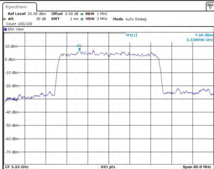
11AX40SISO_Ant0_5550
