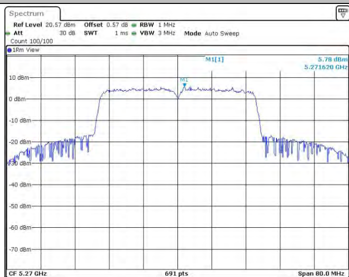
11N40SISO_Ant0_5270
