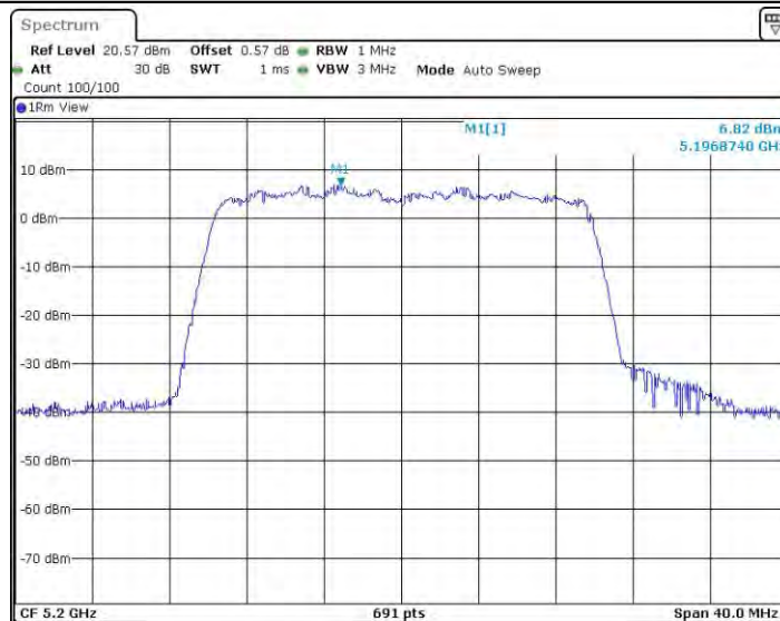
11AX20MIMO_Ant0_5200
