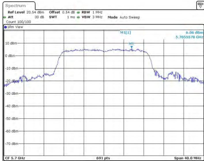
11AC20MIMO_Ant0_5700
