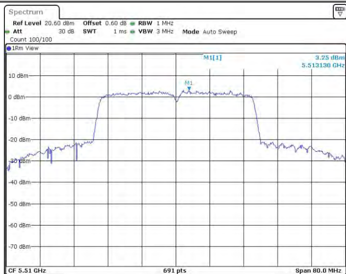
11N40MIMO_Ant0_5510
