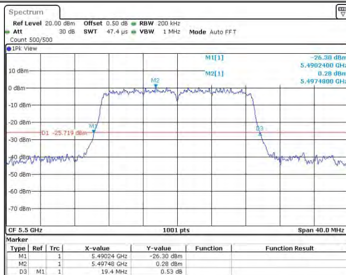
11AC20MIMO_Ant0_5500
