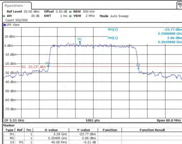
11AX40MIMO_Ant0_5310
