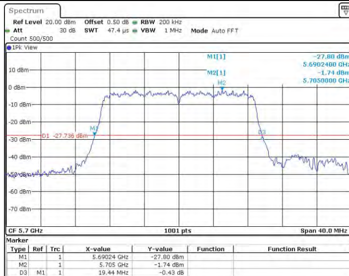
11AC20MIMO_Ant0_5700
