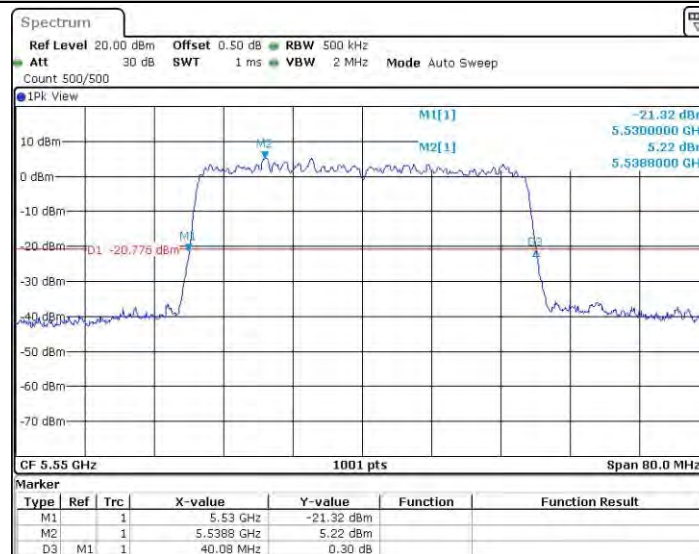
11AX40MIMO_Ant0_5550
