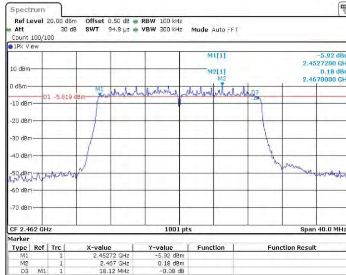
11AX20MIMO_Ant1_2462
