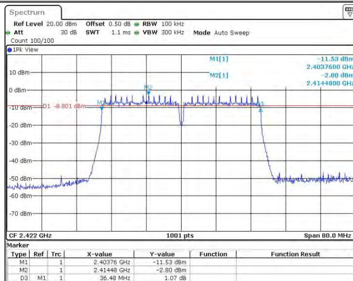
11AC40MIMO_Ant0_2422
