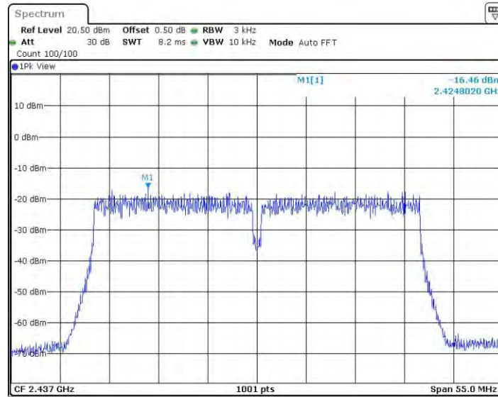
11AC40MIMO_Ant0_2437
