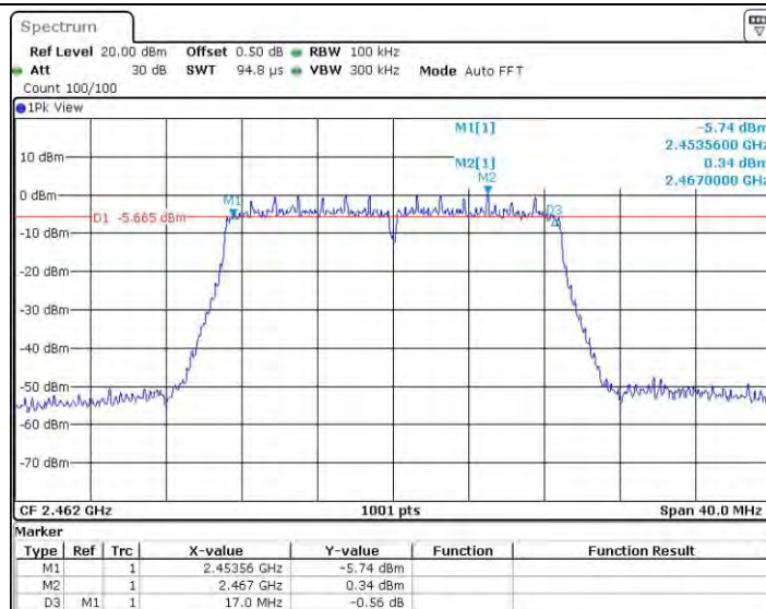
11AC20MIMO_Ant1_2462
