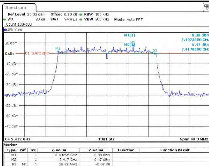
11AX20SISO_Ant0_2412
