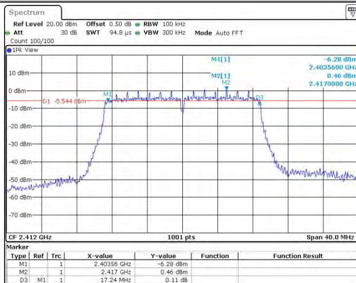
11AC20MIMO_Ant0_2412
