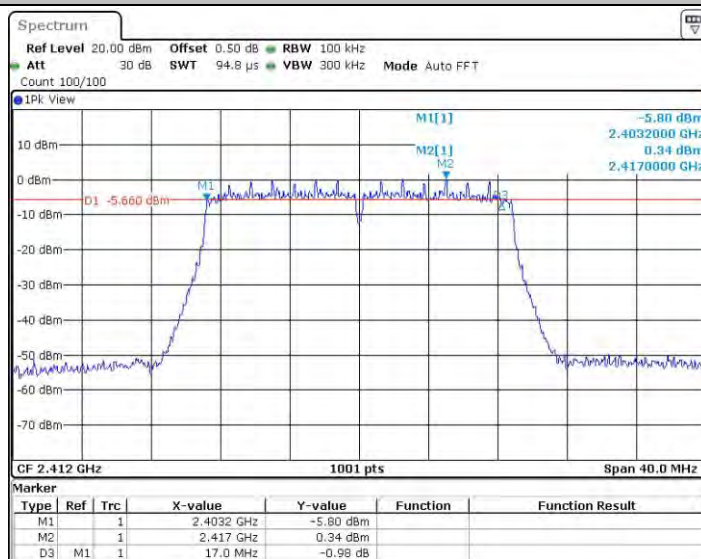
11N20MIMO_Ant0_2412
