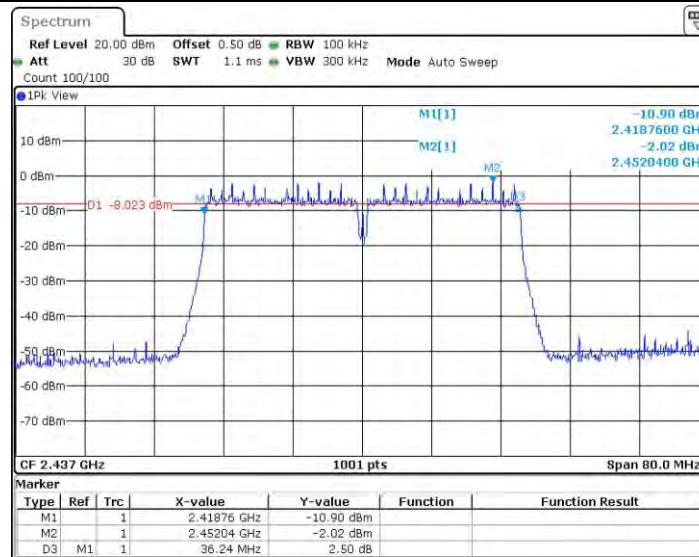
11AC40MIMO_Ant1_2437
