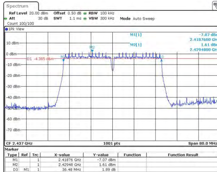
11AC40SISO_Ant0_2437
