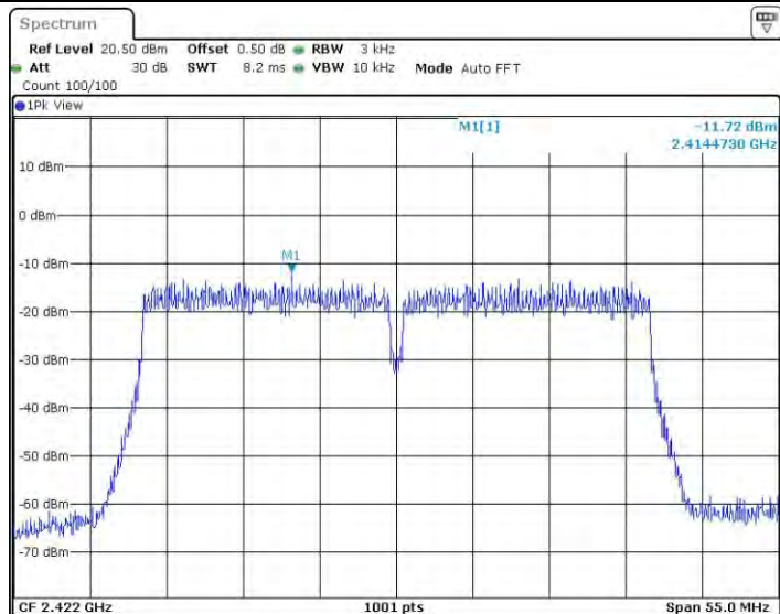
11N40SISO_Ant0_2422
