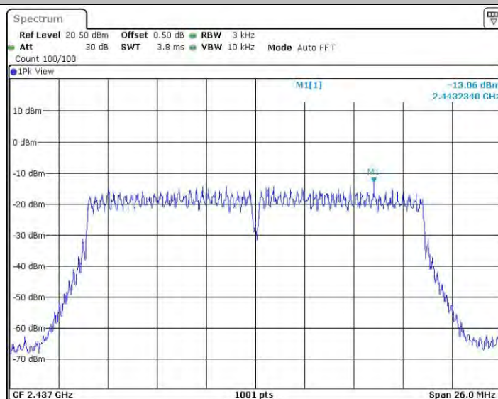
11AC20MIMO_Ant0_2437
