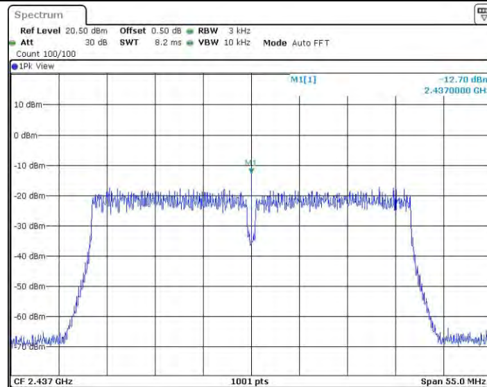
11AC40MIMO_Ant1_2437
