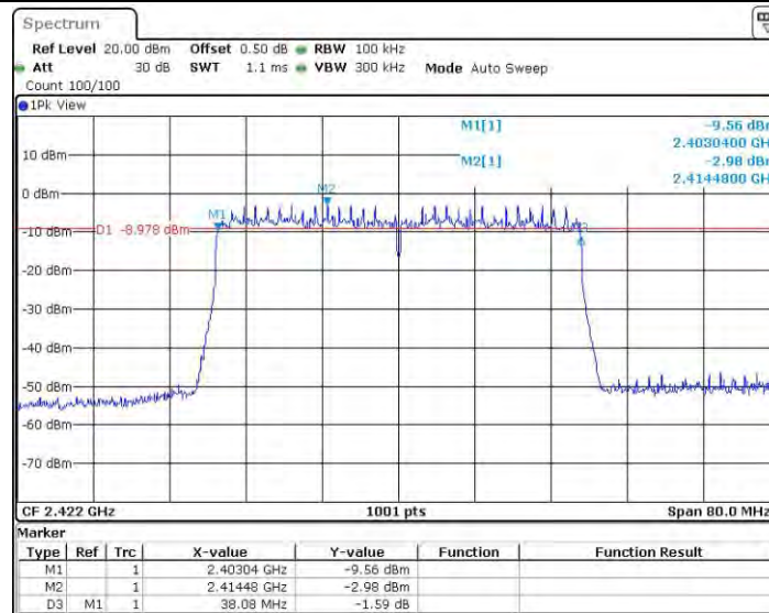
11AX40MIMO_Ant0_2422
