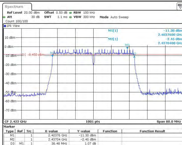
11AC40MIMO_Ant1_2422
