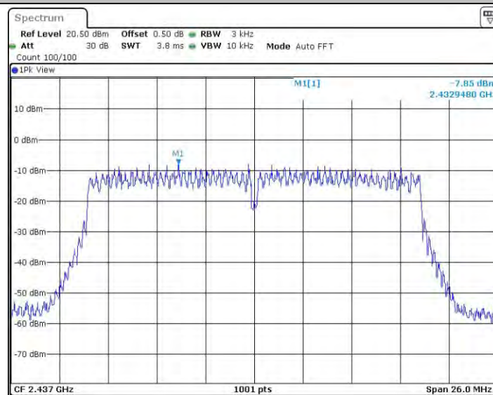
11N20SISO_Ant0_2437
