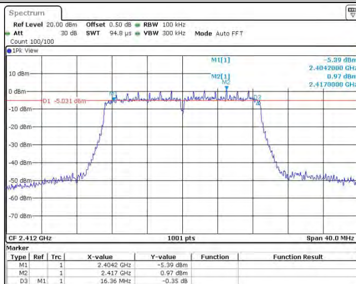
11AC20MIMO_Ant1_2412
