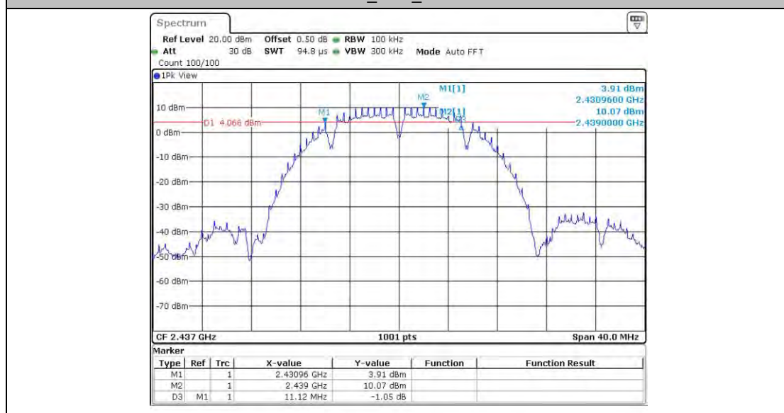
11B_Ant0_2437
