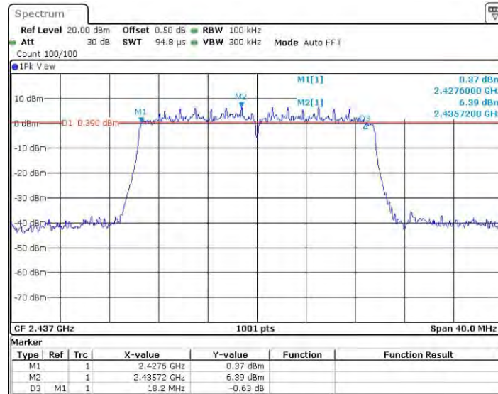
11AX20SISO_Ant0_2437
