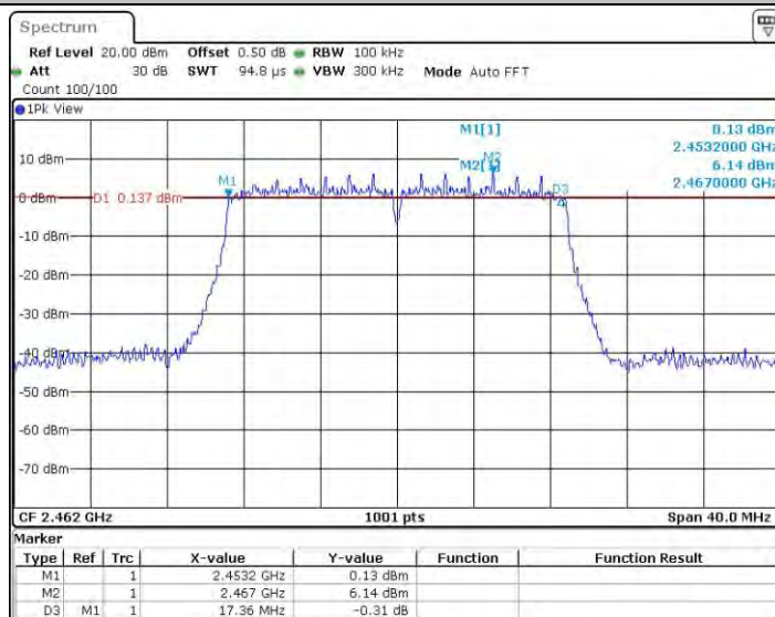
11N20SISO_Ant0_2462
