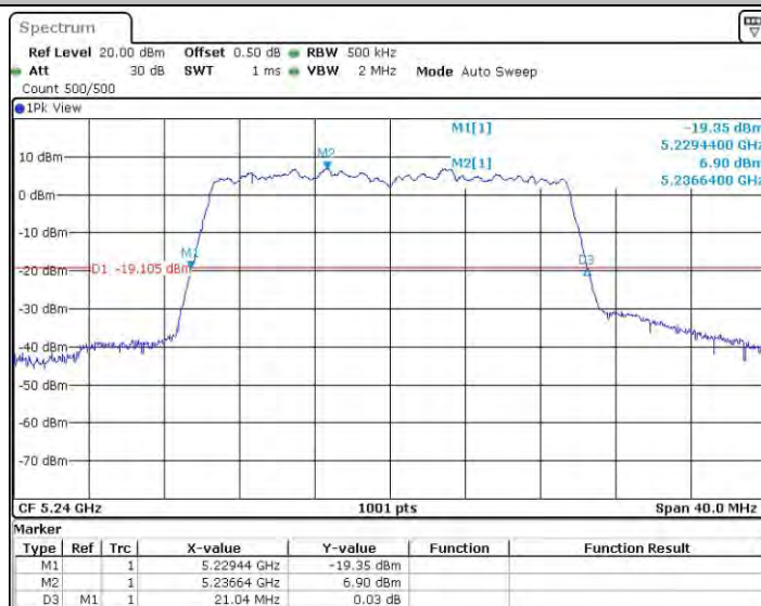
11AX20MIMO_Ant1_5240
