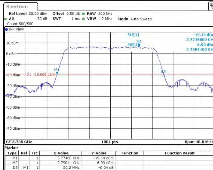
11AC20MIMO_Ant0_5785
