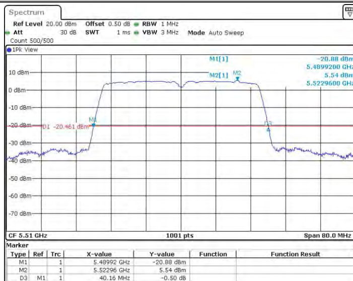
11AC40MIMO_Ant0_5510
