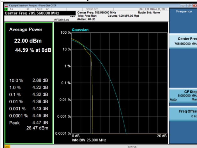
16QAM-23790
