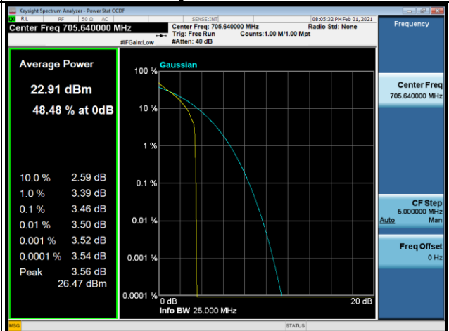
16QAM-23780
