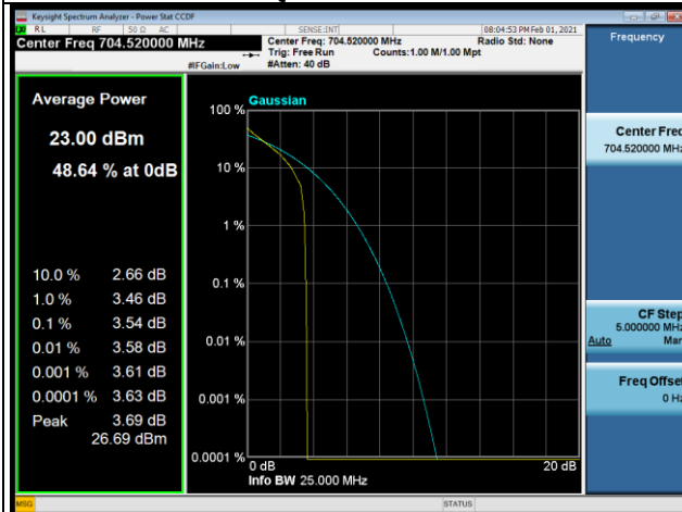
QPSK-23800
