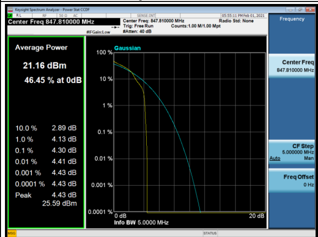
16QAM-20643
