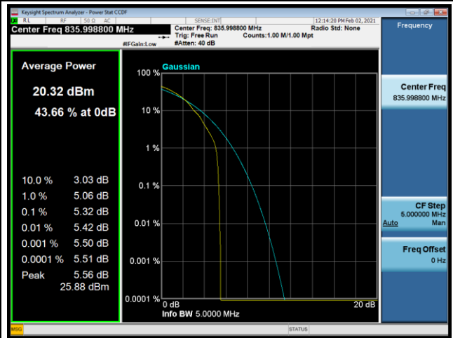
64QAM-20525
