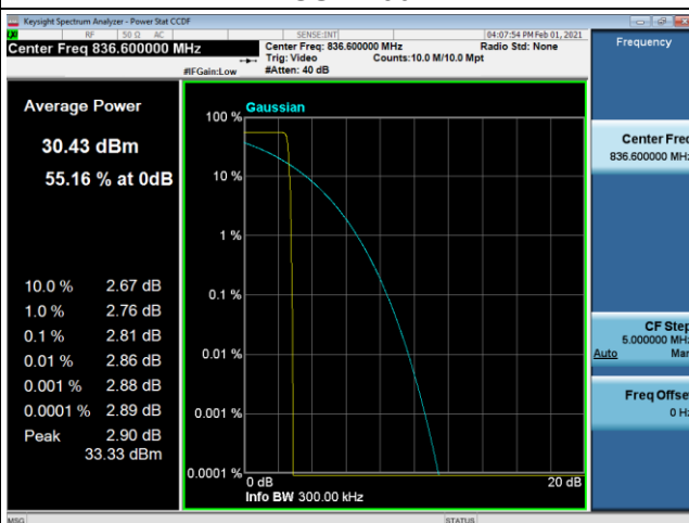
EDGE-128
