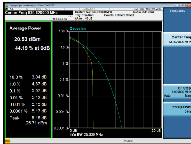
64QAM-20600
