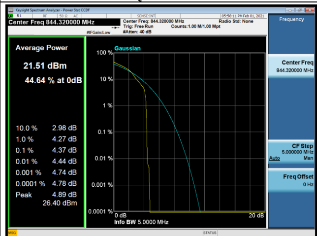
16QAM-20625
