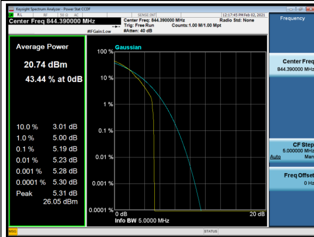
64QAM-20625
