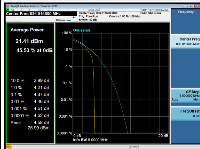
16QAM-20525
