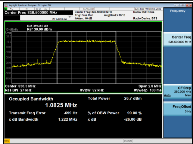
64QAM-20525
