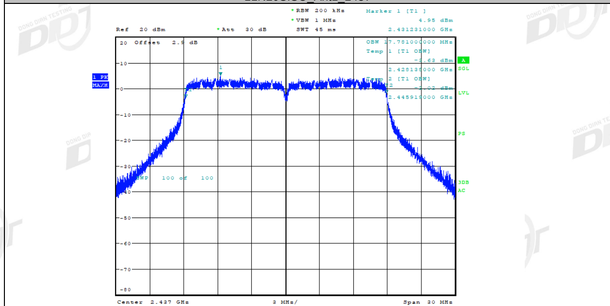
11N20SISO_Ant1_2437
