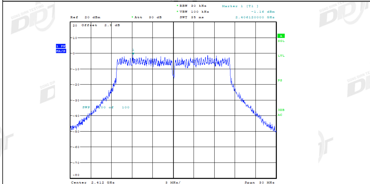
11G_Ant1_2412
