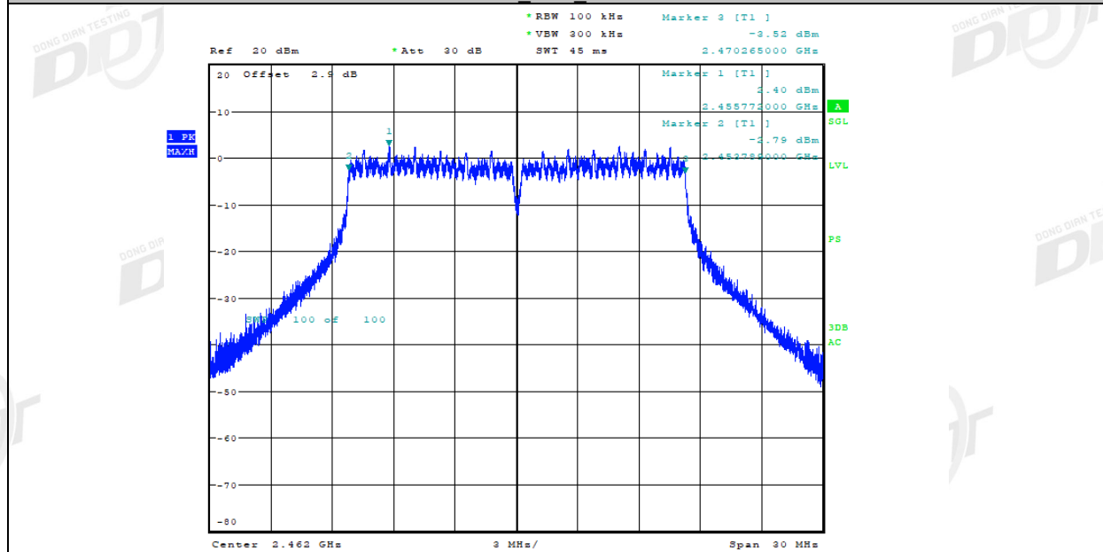
11G_Ant1_2462
