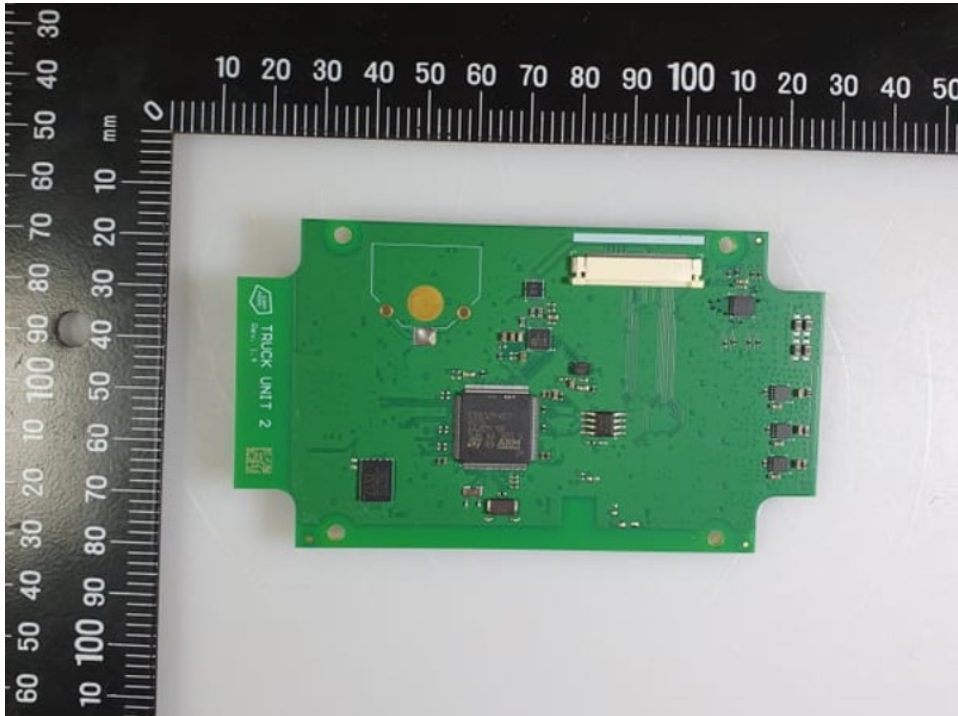
Photo 3: EUT 1
