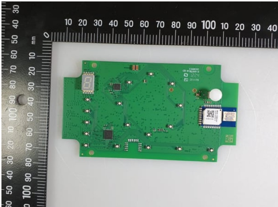
Photo 4: EUT 1
