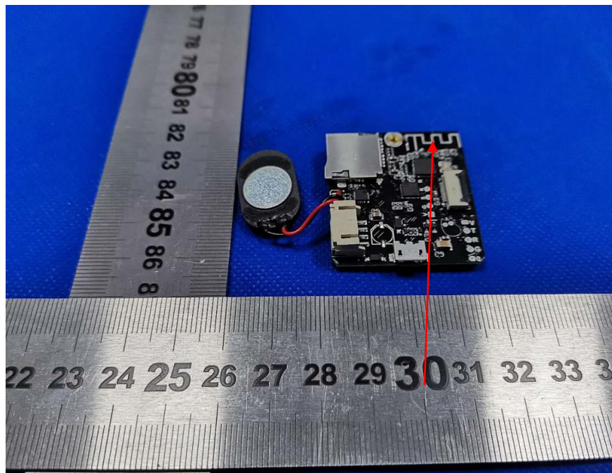
Antenna
