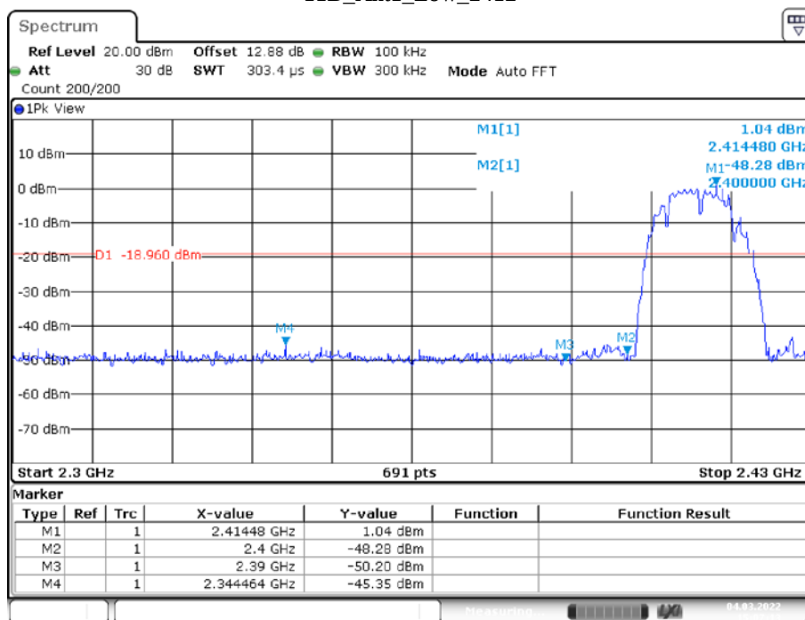
11B_Ant1_Low_2412
