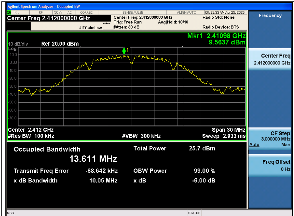
Test_Graph_802.11b_ANT1_2412_1Mbps_DTSSBW
