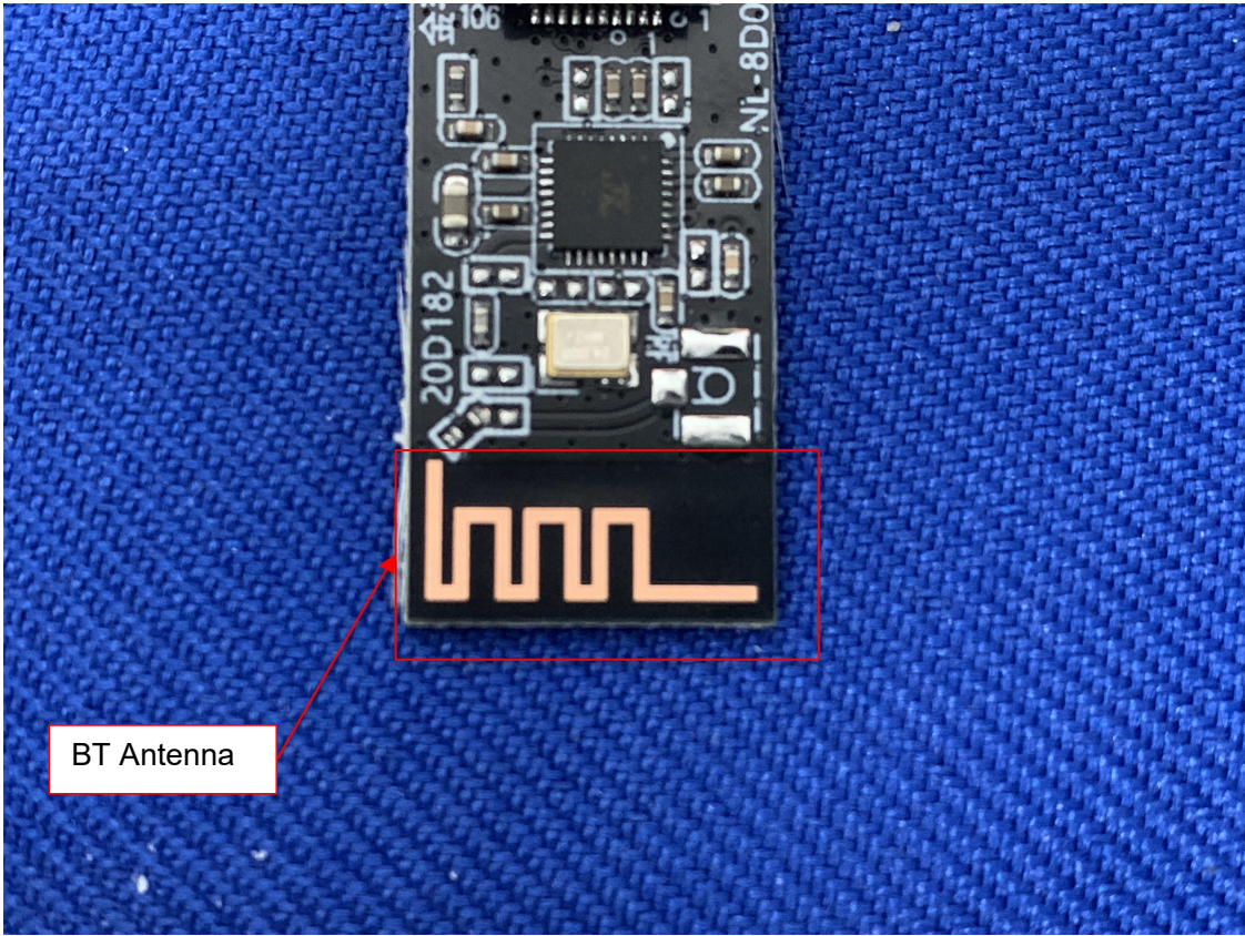
EUT Photo
