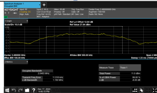
BLE 2M_Channel 39
