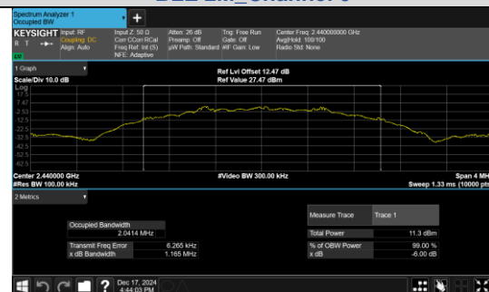
BLE 2M_Channel 19
