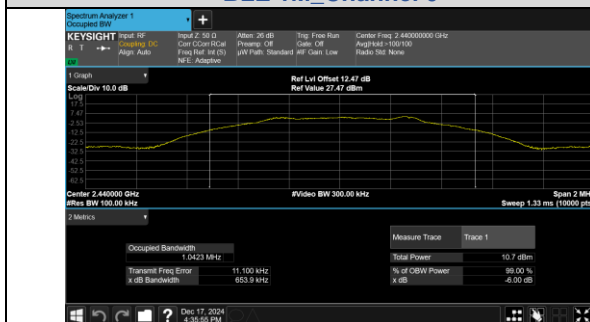
BLE 1M_Channel 19
