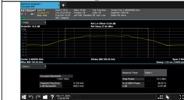
BLE 1M_Channel 39
