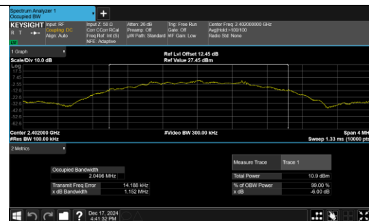
BLE 2M_Channel 0
