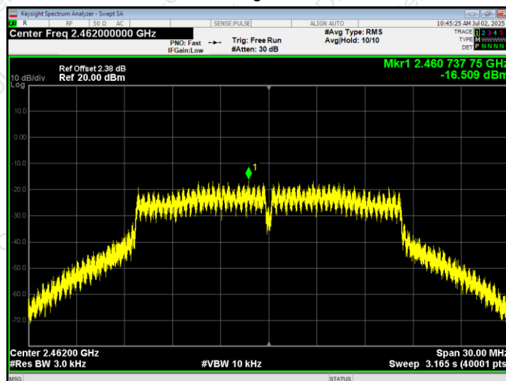
802.11g - CH11
