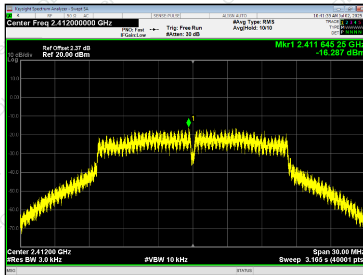
802.11g - CH01
