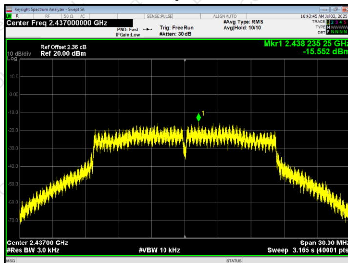
802.11g - CH06
