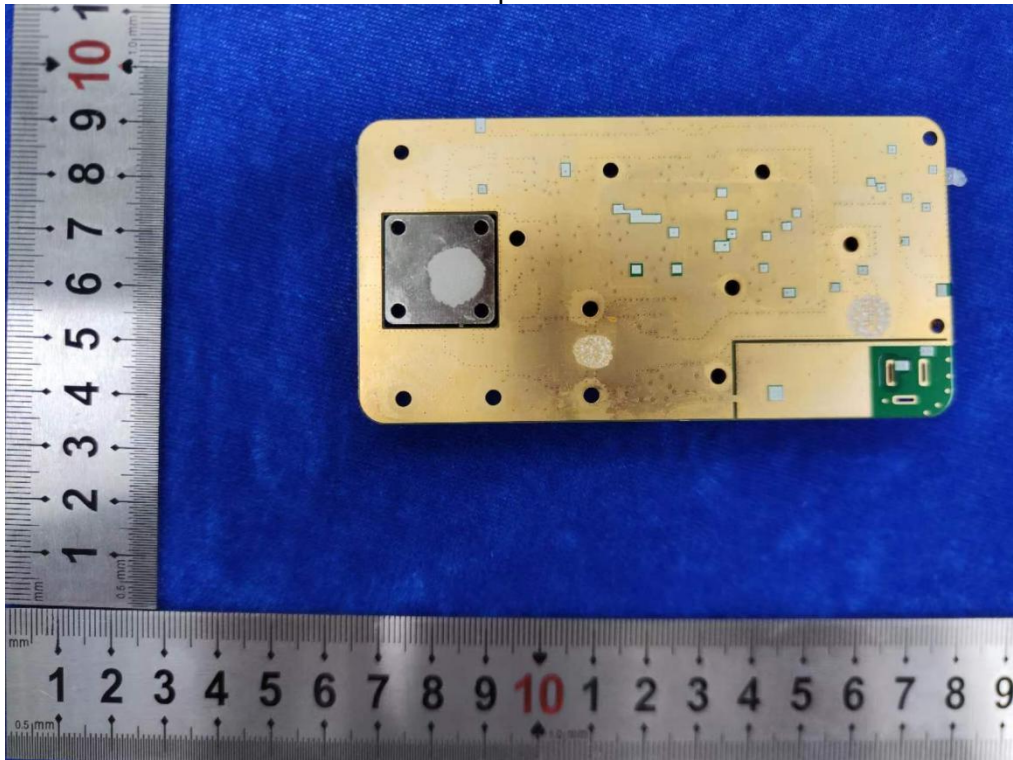
EUT photo3
