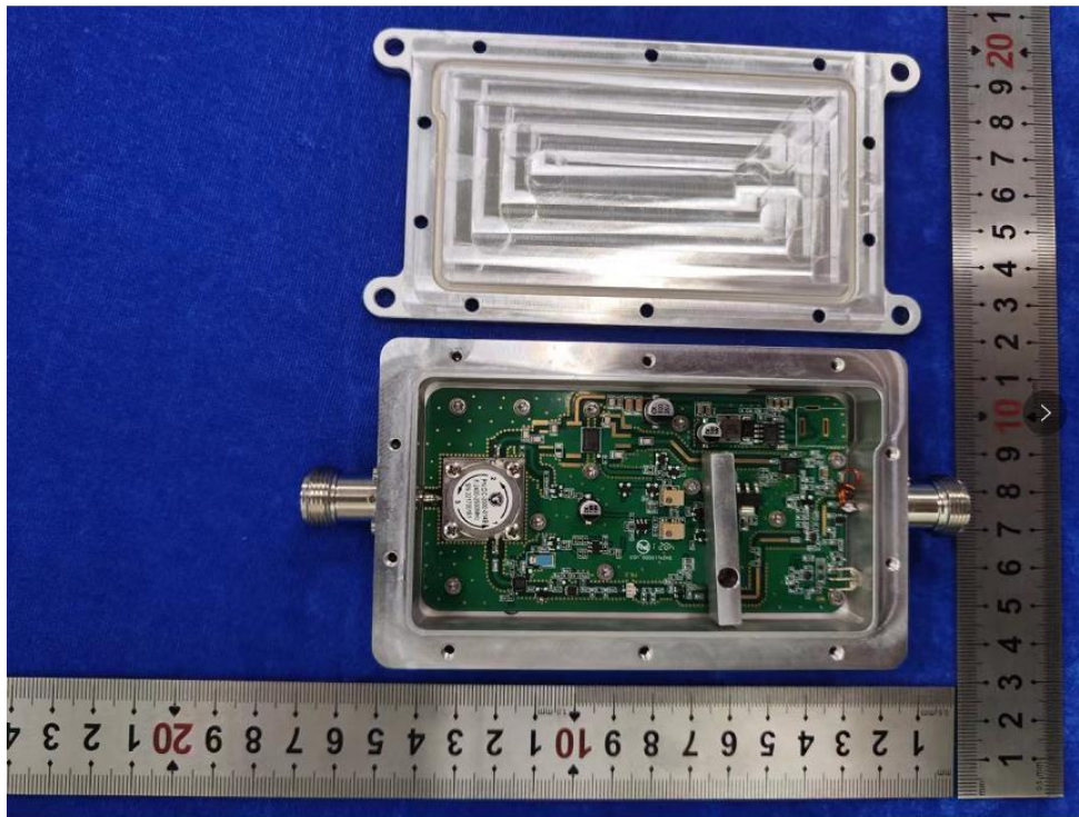
EUT photo2
