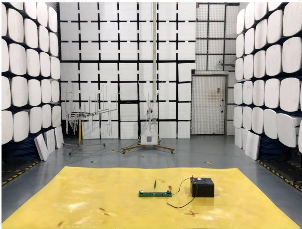
Fig. 1 (2.4G WLAN)
