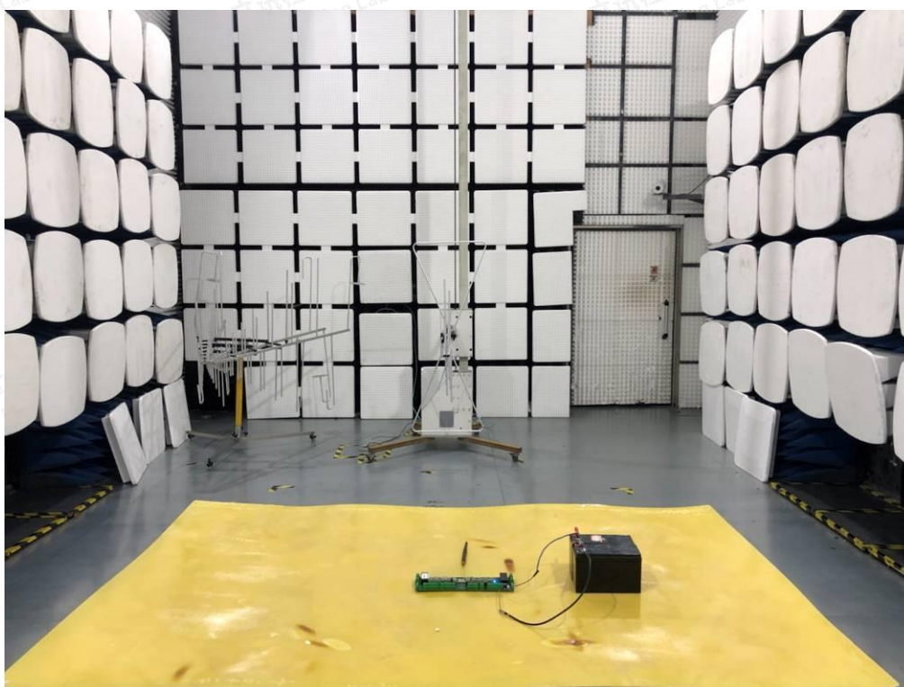
Fig. 3 (433M)
