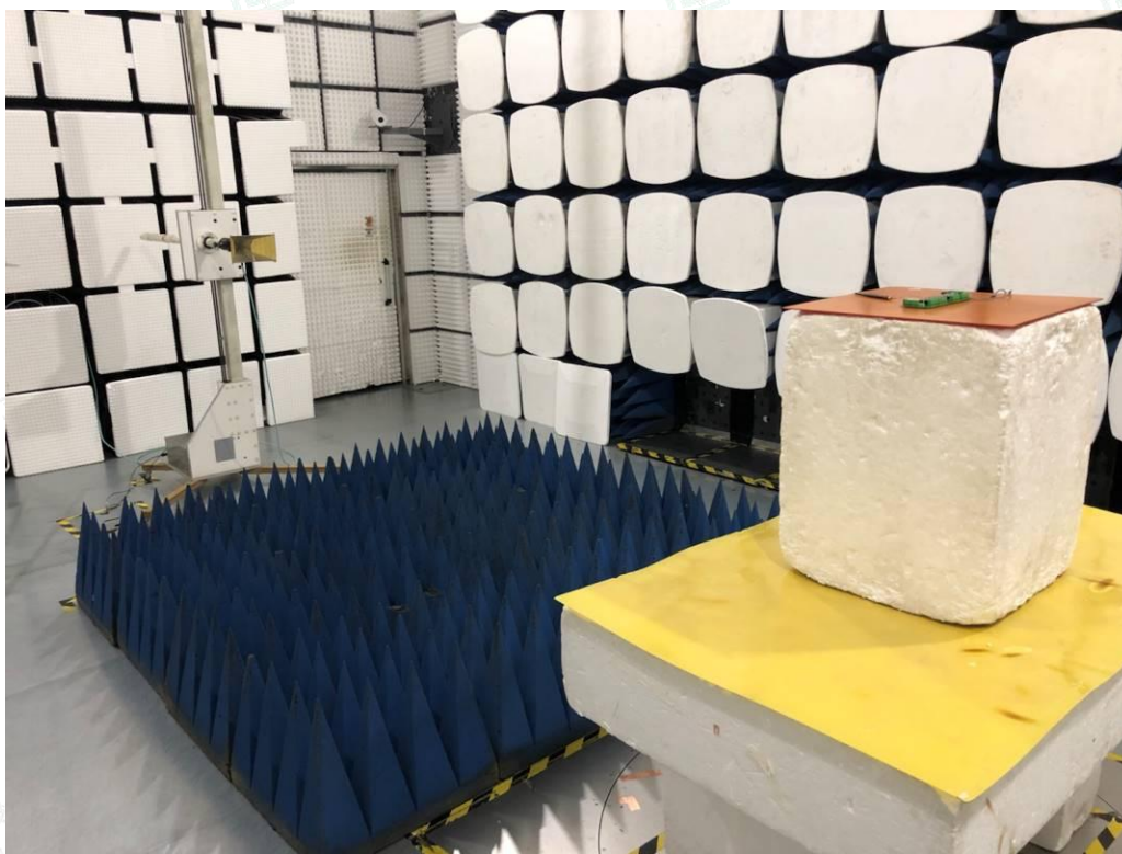
Fig. 2 (2.4G WLAN)
