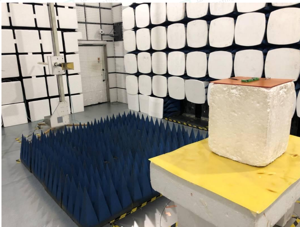
Fig. 4 (433M)
