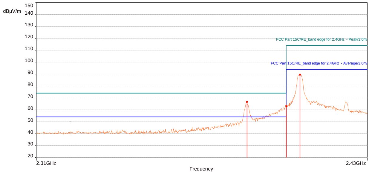
2405MHz Vertical
