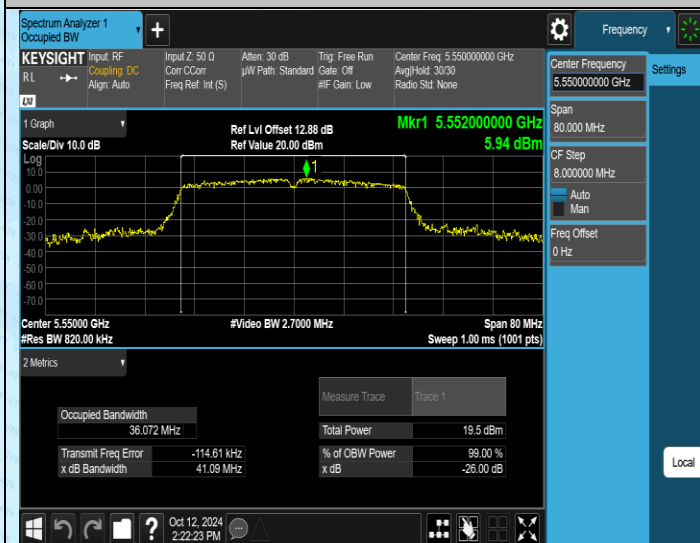
11AC40MIMO-Ant1-5550
