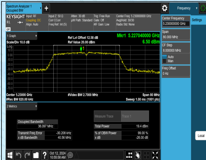
11N40MIMO-Ant1-5230
