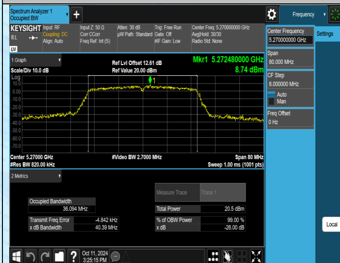
11N40SISO-Ant1-5270
