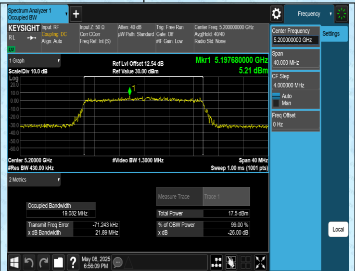
11AX20SISO-Ant1-5200
