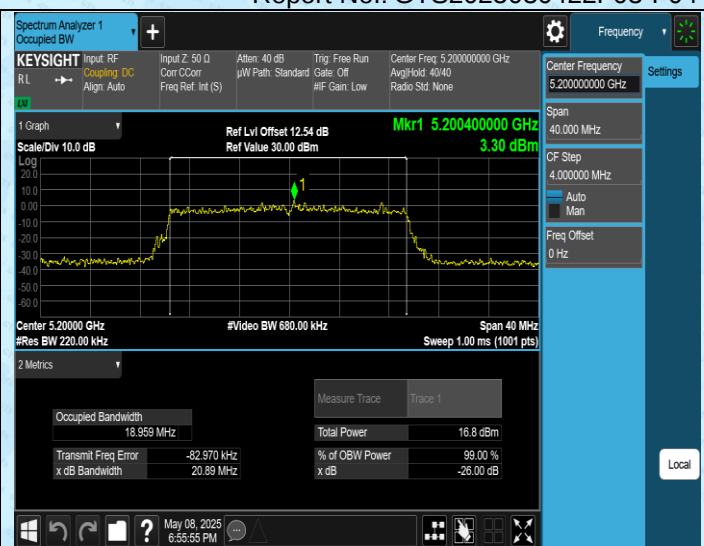
11AX20SISO-Ant1-5200
