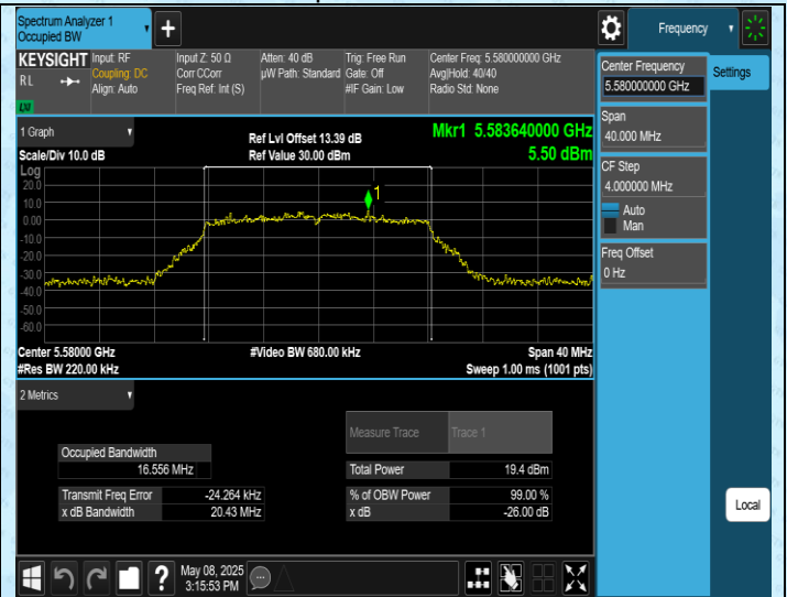
11A-Ant1-5580
