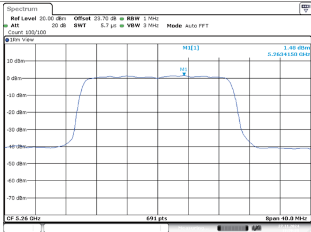
11AX20MIMO-Ant1-5260-PASS
