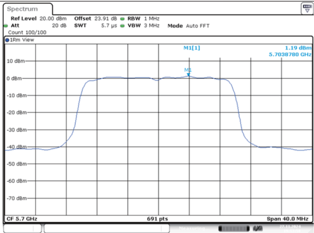
11AX20MIMO-Ant1-5700-PASS
