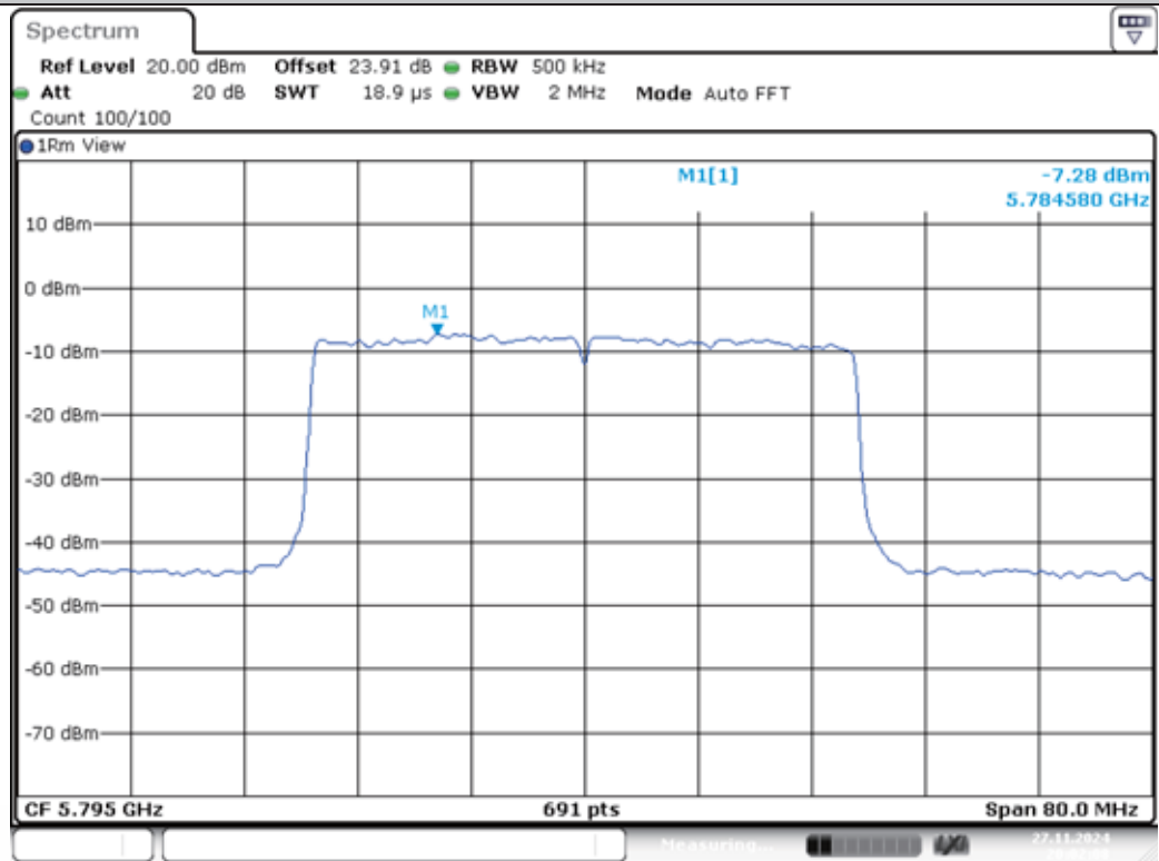
11AX40MIMO-Ant1-5795-PASS
