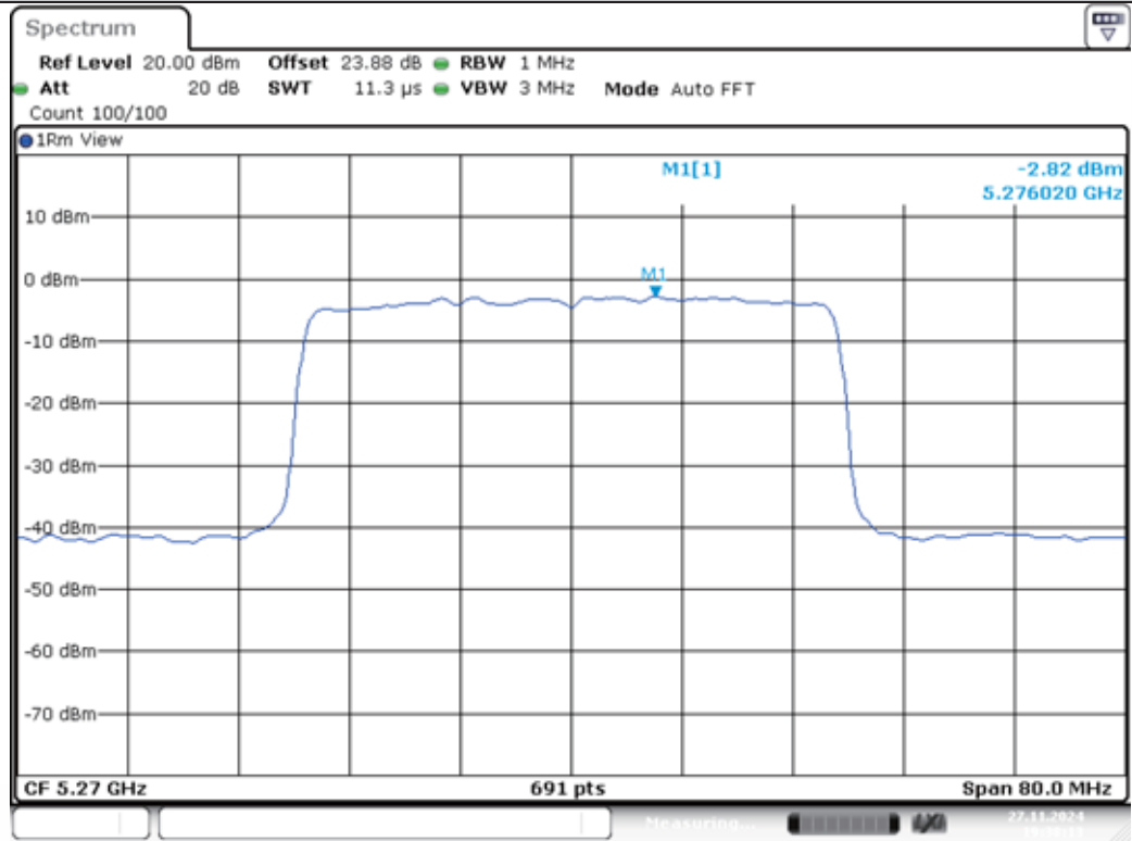
11AX40MIMO-Ant1-5270-PASS
