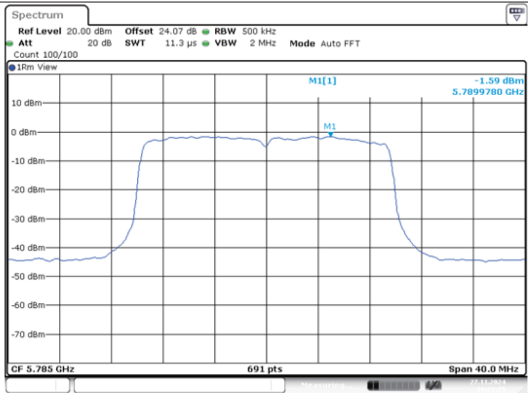
11AX20MIMO-Ant1-5785-PASS
