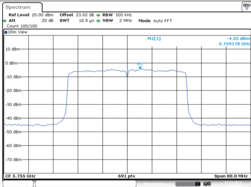
11AX40MIMO-Ant1-5755-PASS
