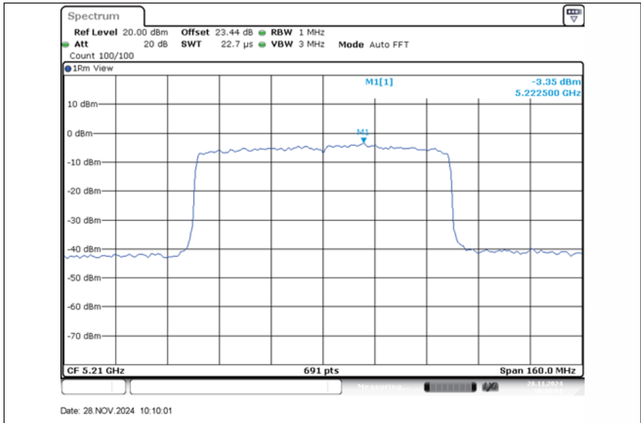
11AX80MIMO-Ant1-5210-PASS
