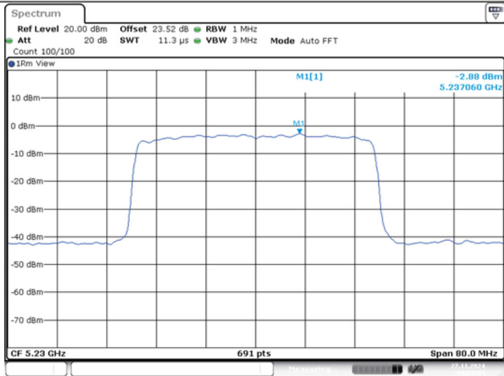
11AX40MIMO-Ant1-5230-PASS
