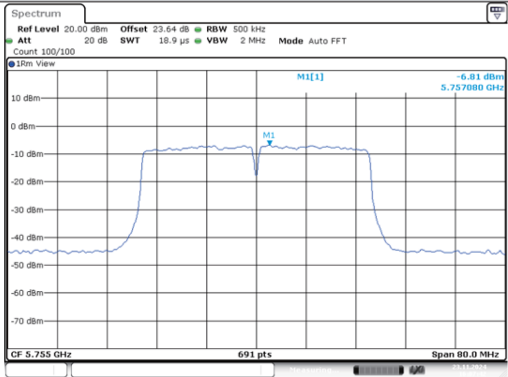
11N40MIMO-Ant1-5755-PASS
