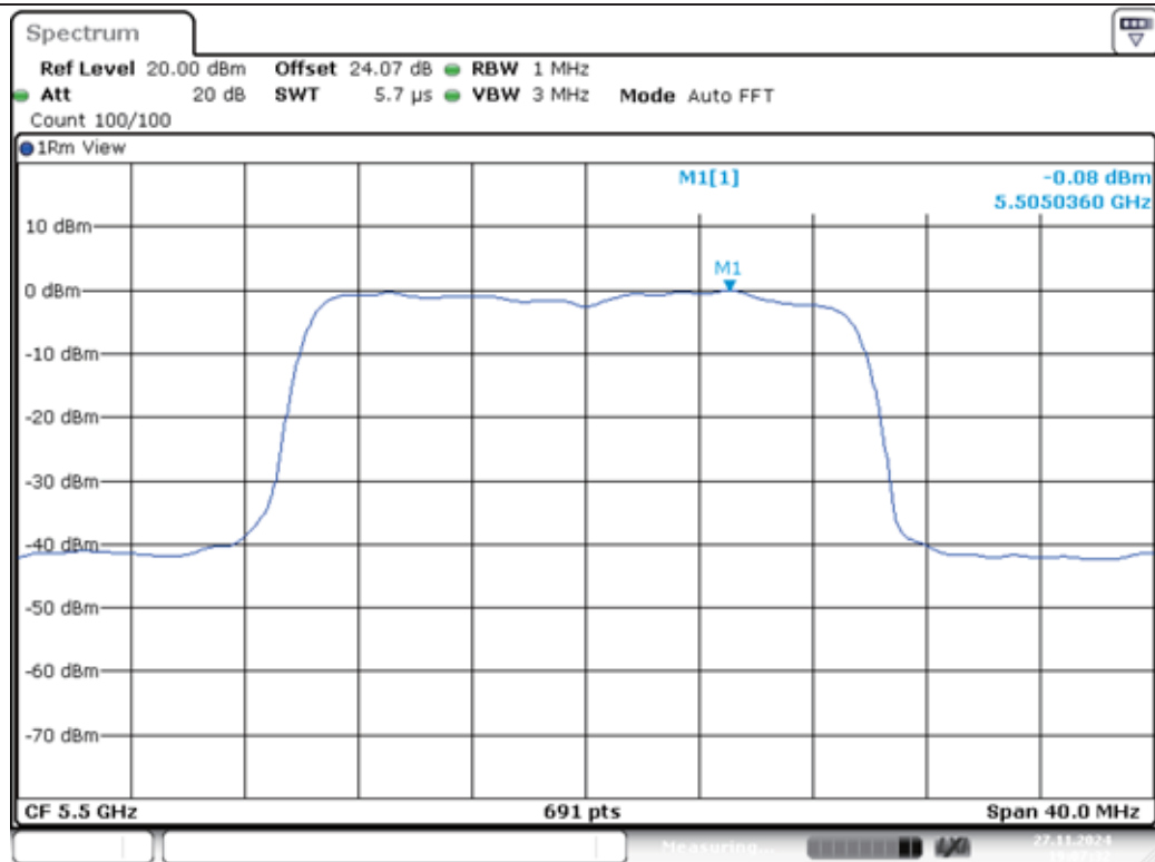
11AX20MIMO-Ant1-5500-PASS
