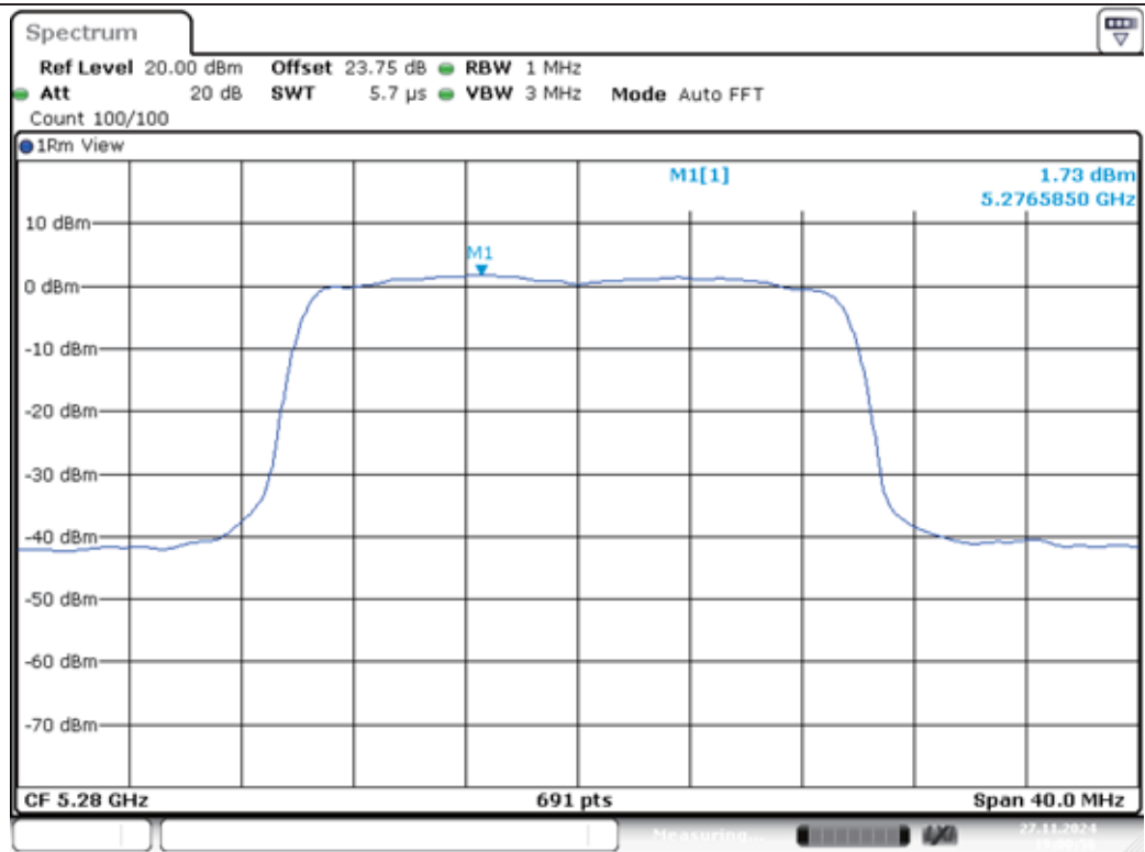
11AX20MIMO-Ant1-5280-PASS
