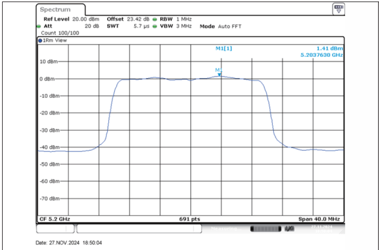
11AX20MIMO-Ant1-5200-PASS
