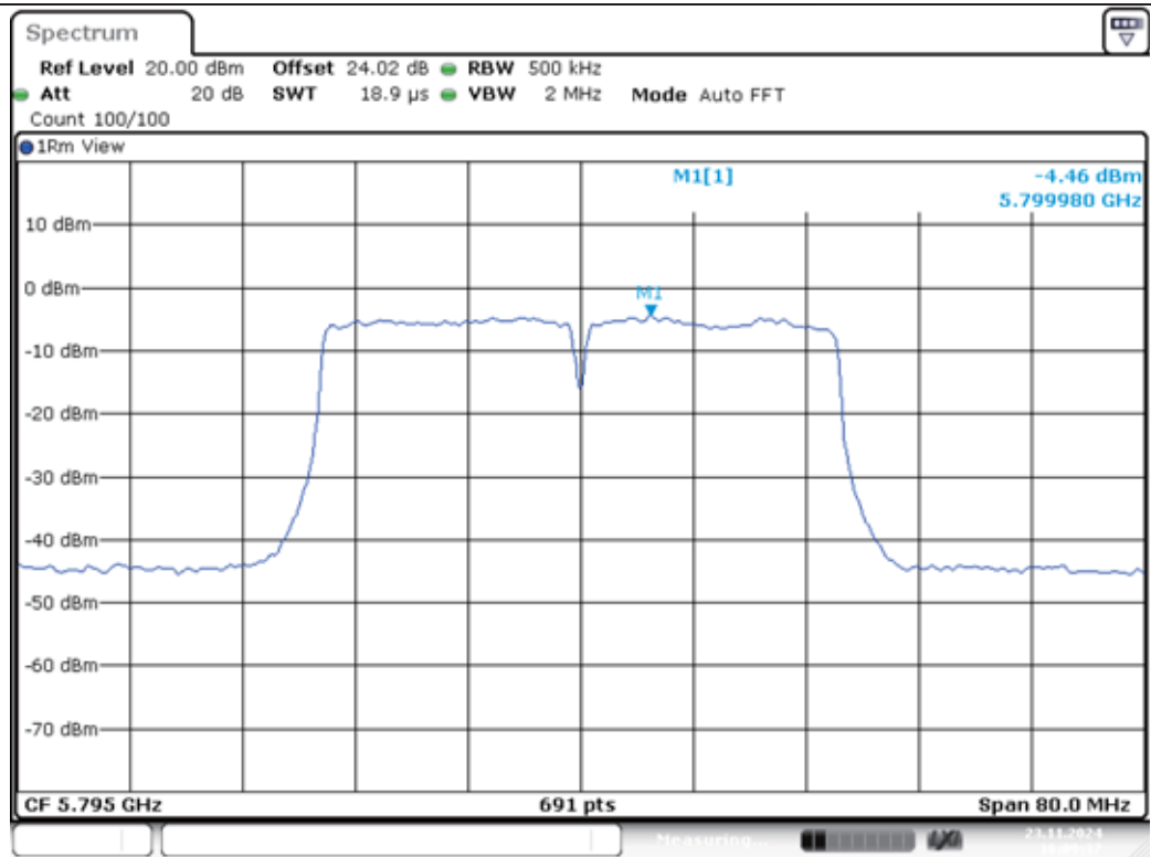
11N40MIMO-Ant1-5795-PASS
