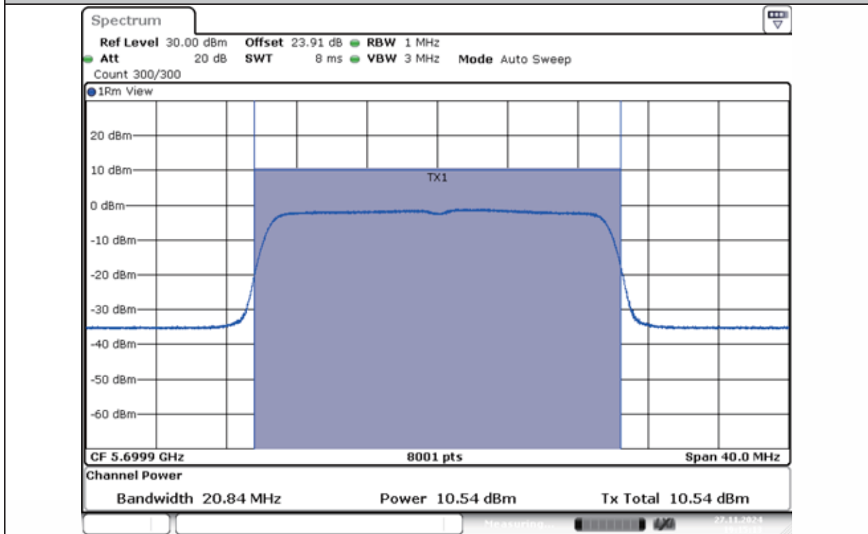
11AX20MIMO-Ant1-5700-PASS
