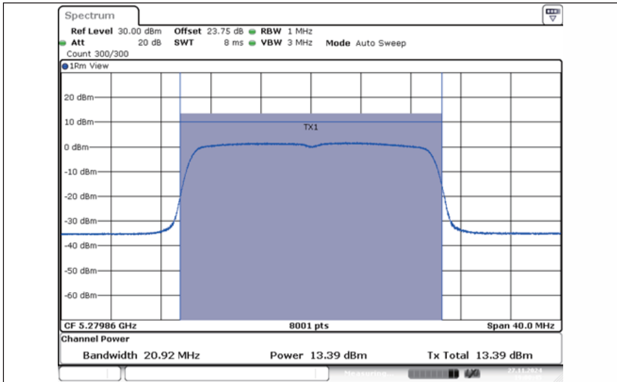
11AX20MIMO-Ant1-5280-PASS
