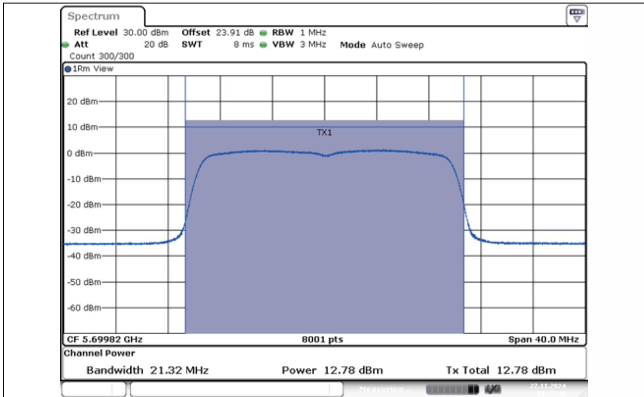
11AX20MIMO-Ant1-5700-PASS
