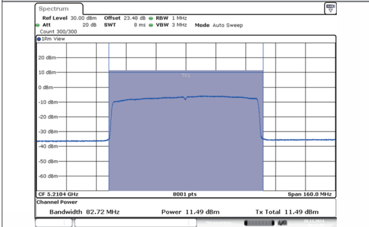
11AX80MIMO-Ant1-5210-PASS
