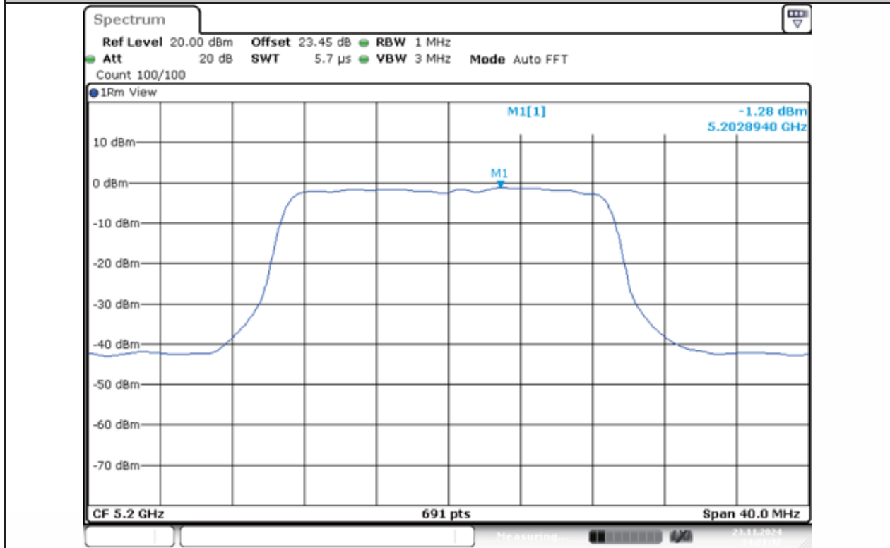
11N20MIMO-Ant1-5200-PASS
