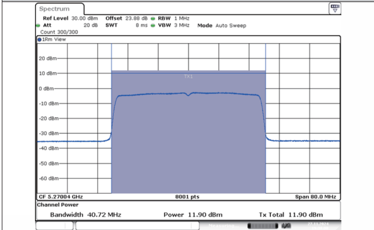
11AX40MIMO-Ant1-5270-PASS
