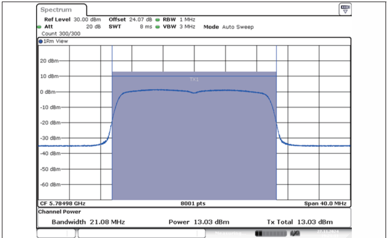
11AX20MIMO-Ant1-5785-PASS
