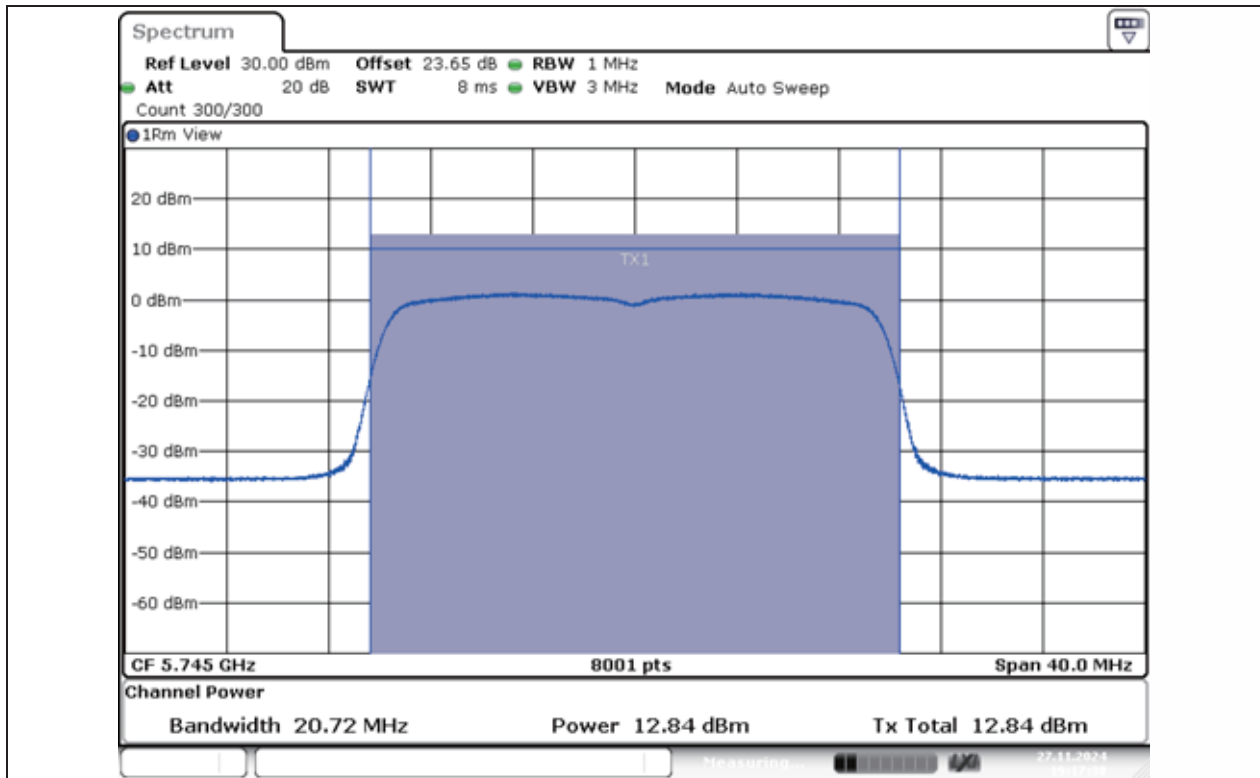
11AX20MIMO-Ant1-5745-PASS
