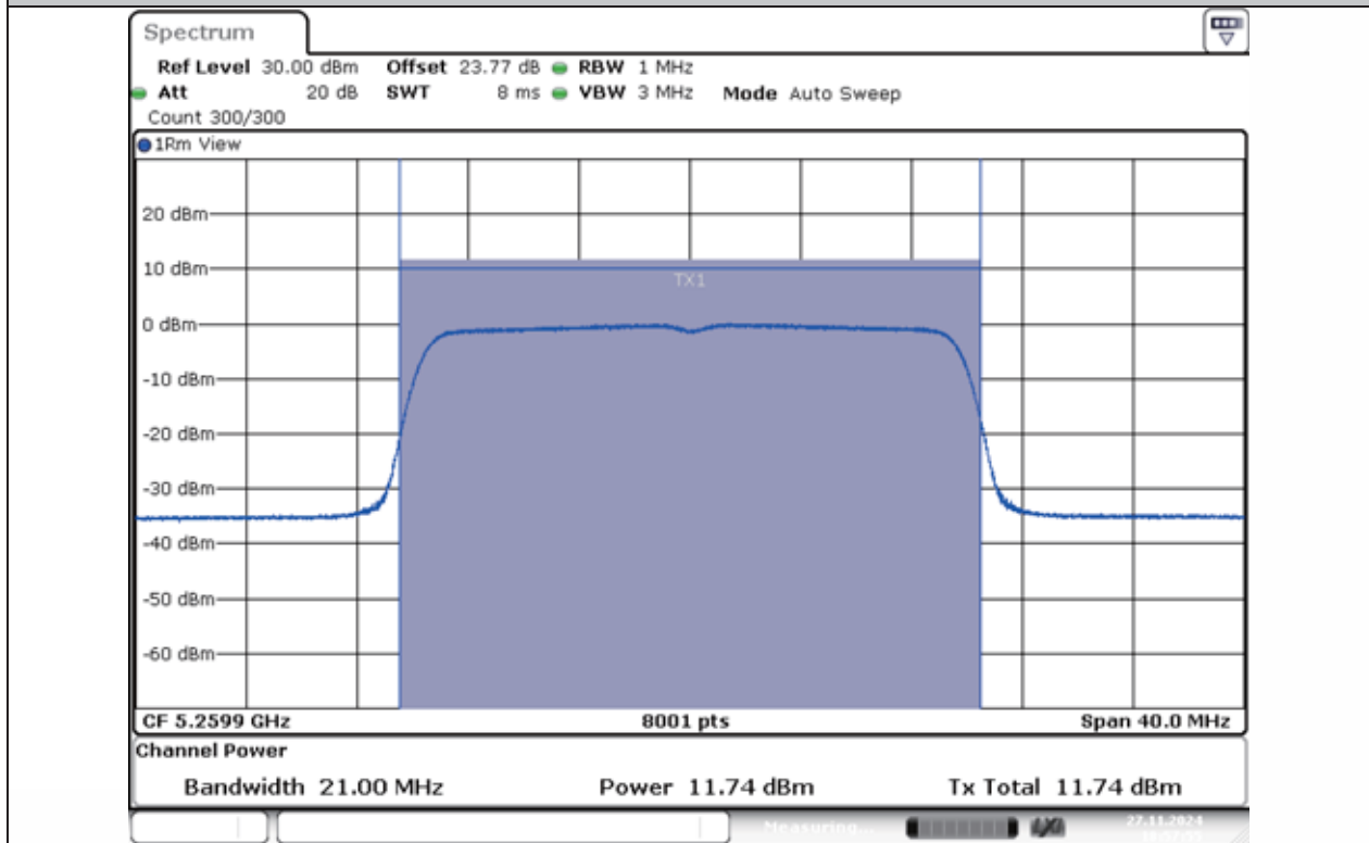
11AX20MIMO-Ant1-5260-PASS
