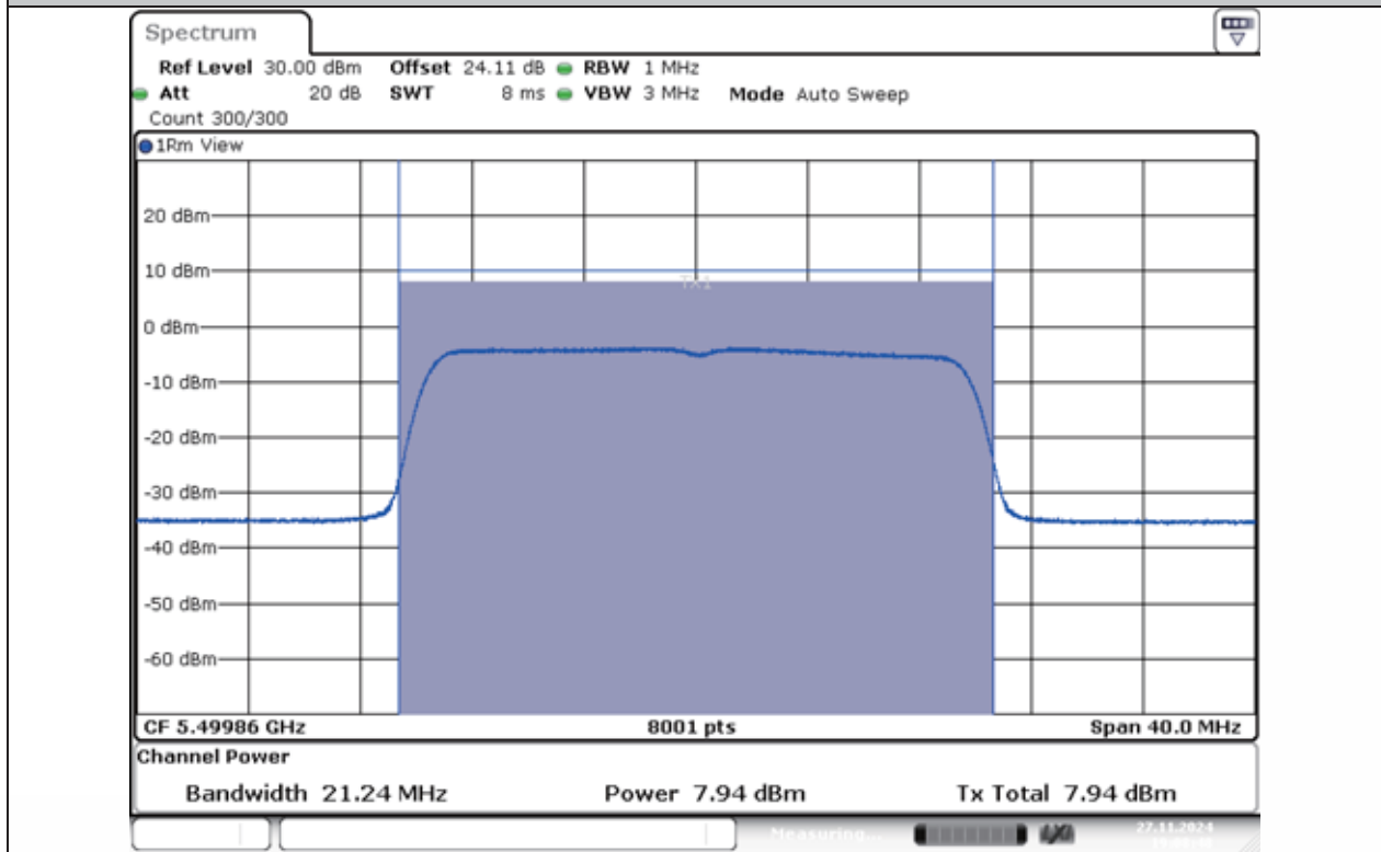
11AX20MIMO-Ant1-5500-PASS
