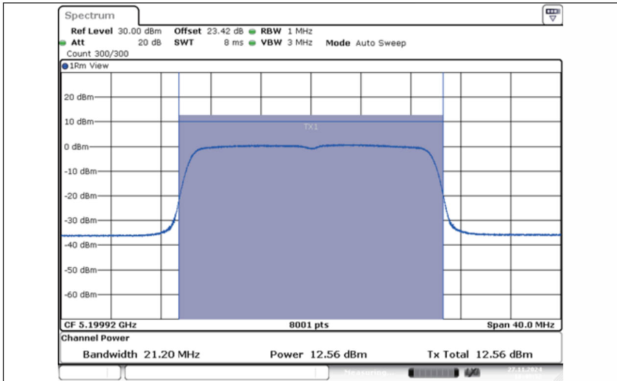
11AX20MIMO-Ant1-5200-PASS
