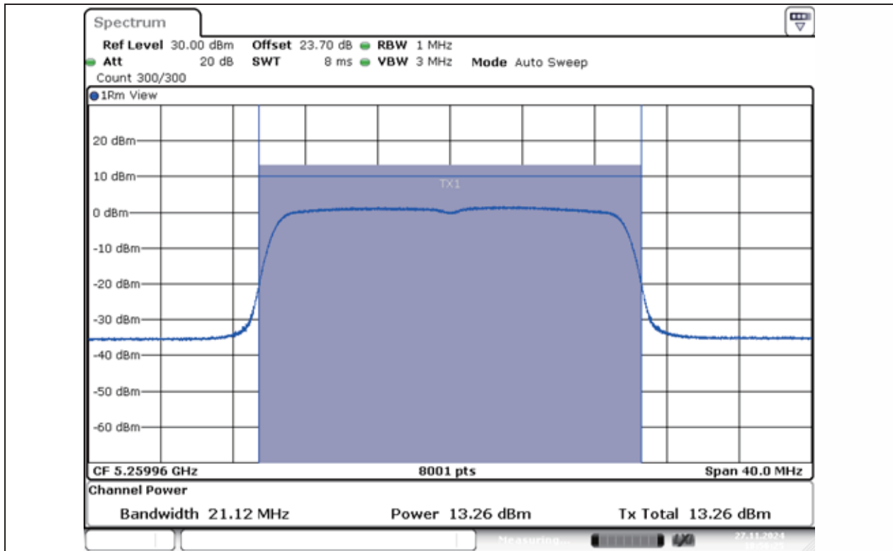
11AX20MIMO-Ant1-5260-PASS
