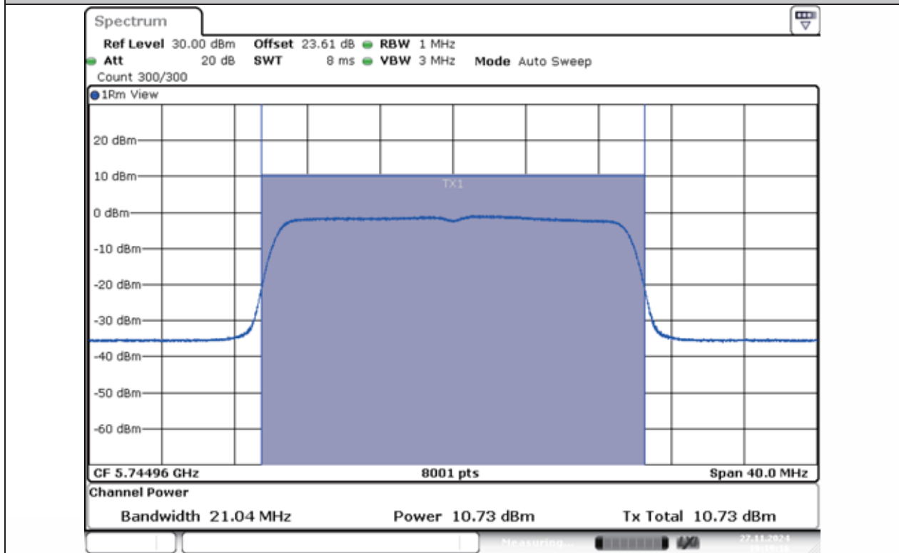
11AX20MIMO-Ant1-5745-PASS
