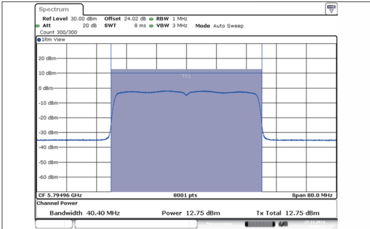
11AX40MIMO-Ant1-5795-PASS
