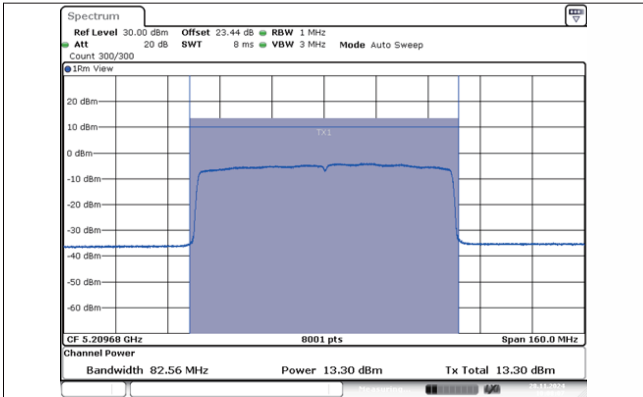
11AX80MIMO-Ant1-5210-PASS
