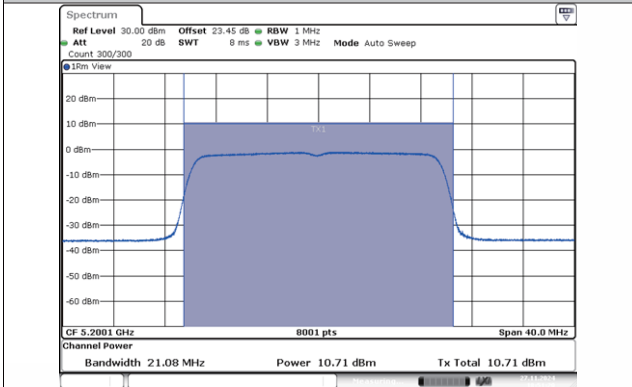
11AX20MIMO-Ant1-5200-PASS
