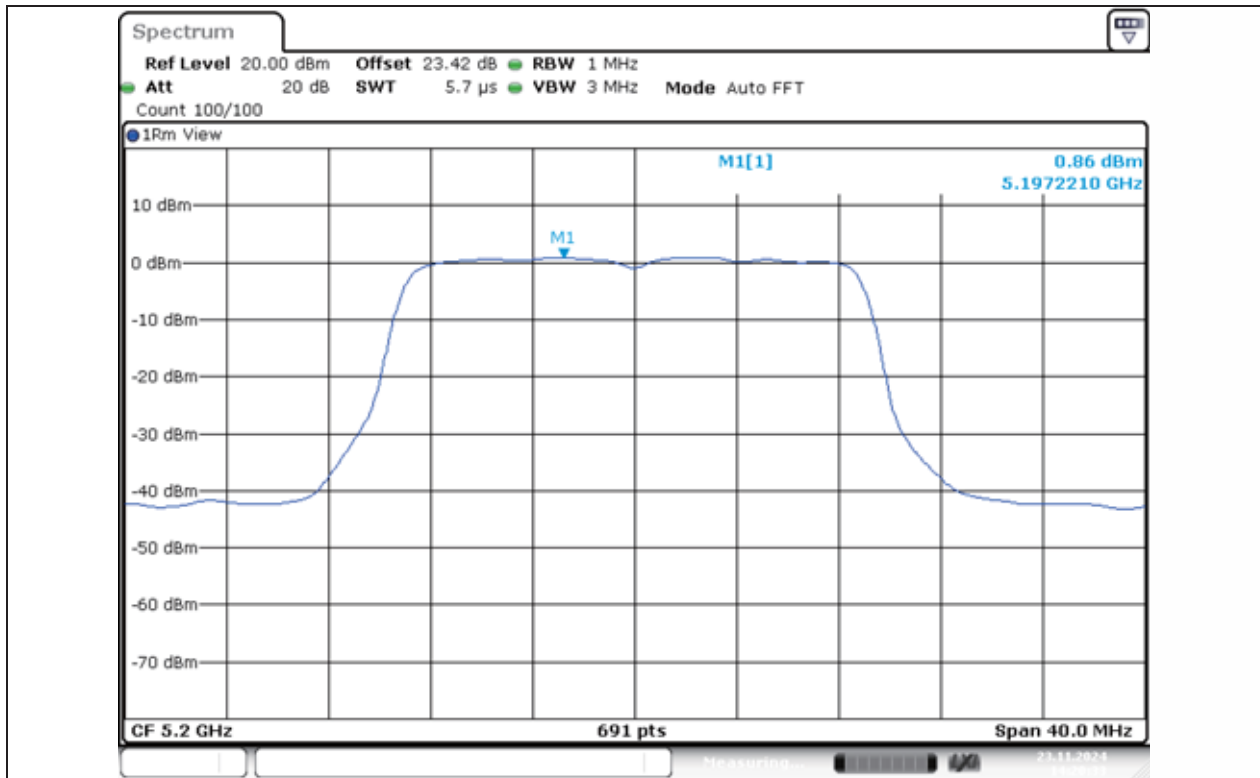
11N20MIMO-Ant1-5200-PASS
