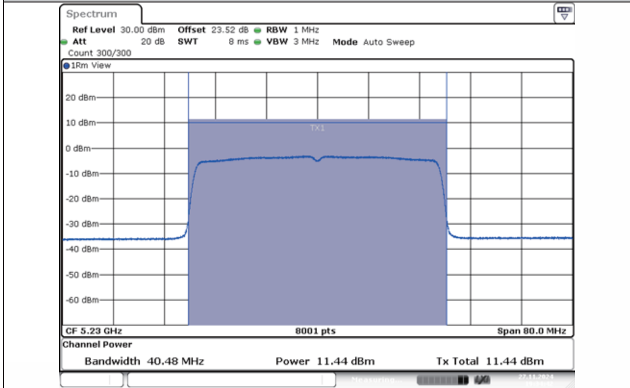
11AX40MIMO-Ant1-5230-PASS
