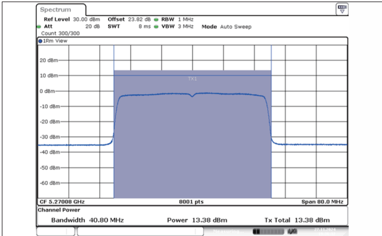
11AX40MIMO-Ant1-5270-PASS
