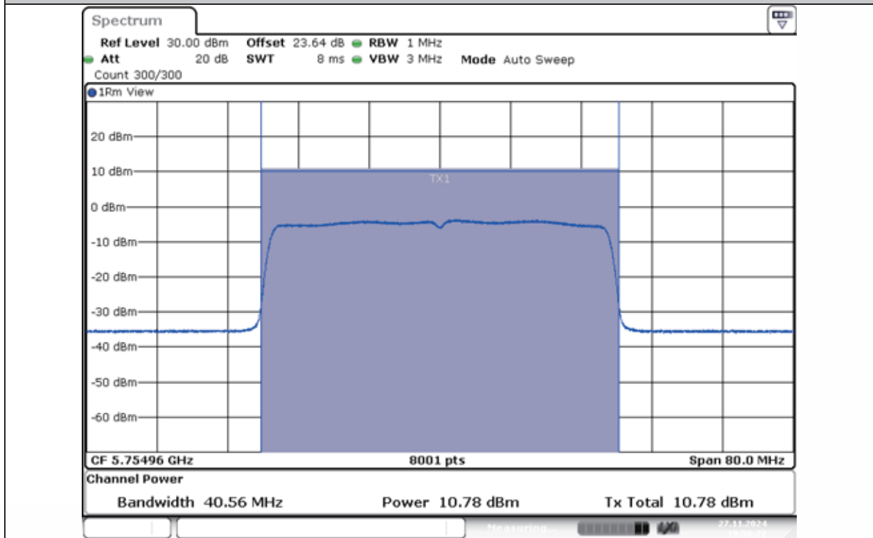
11AX40MIMO-Ant1-5755-PASS
