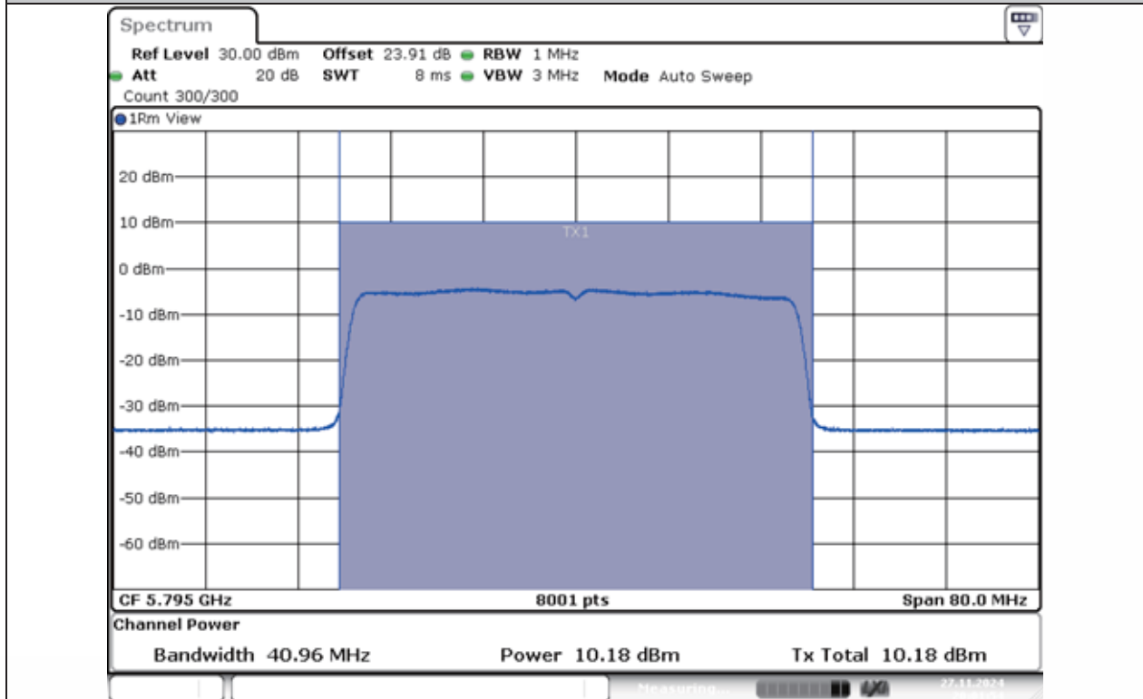
11AX40MIMO-Ant1-5795-PASS
