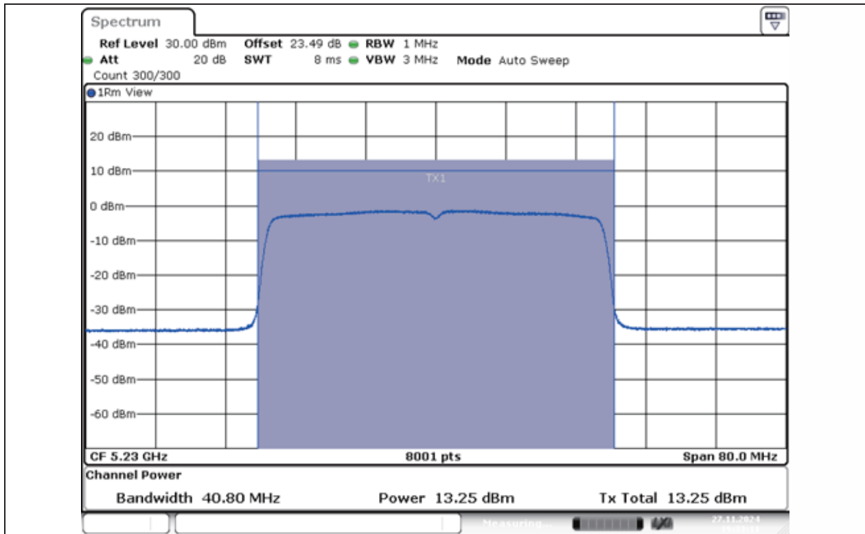
11AX40MIMO-Ant1-5230-PASS
