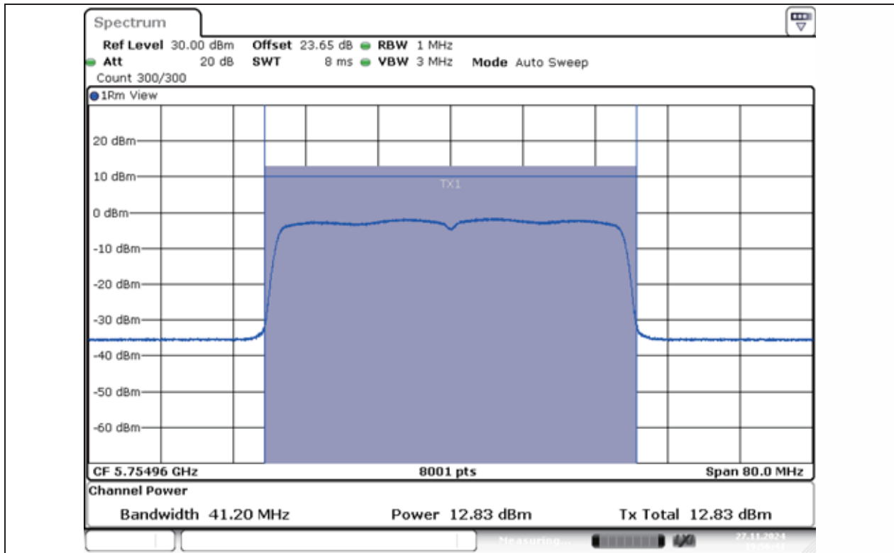
11AX40MIMO-Ant1-5755-PASS
