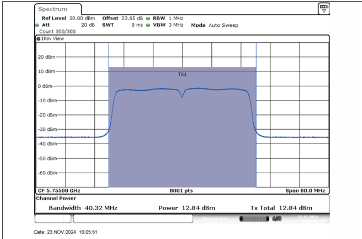
11N40MIMO-Ant1-5755-PASS
