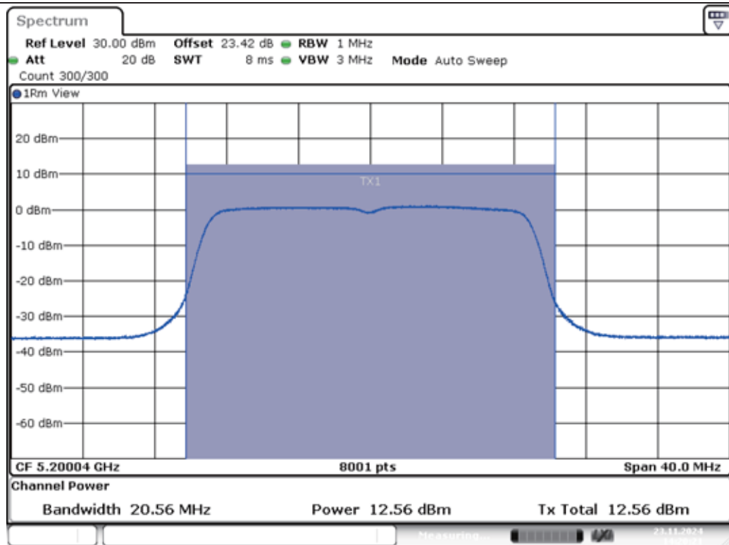
11N20MIMO-Ant1-5200-PASS
