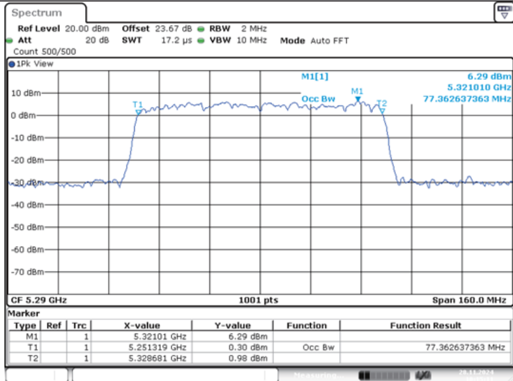
11AX80MIMO-Ant1-5290
