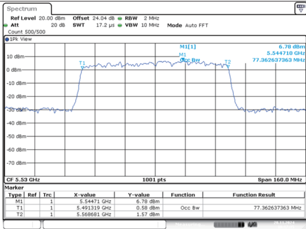
11AX80MIMO-Ant1-5530
