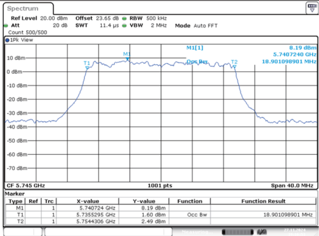
11AX20MIMO-Ant1-5745
