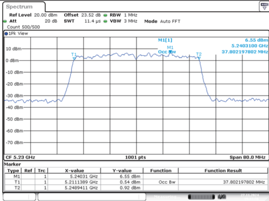
11AX40MIMO-Ant1-5230
