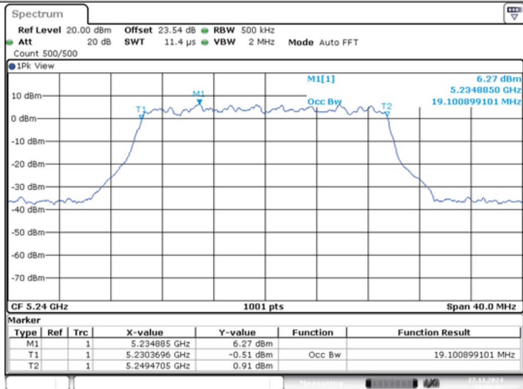
11AX20MIMO-Ant1-5240
