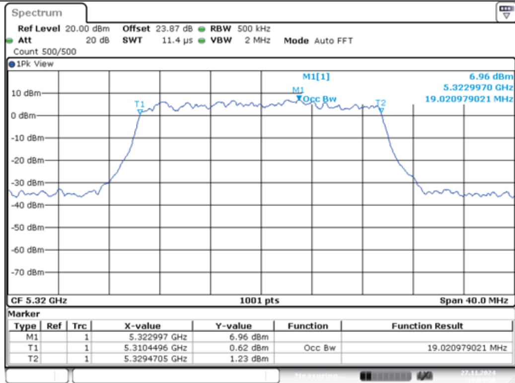
11AX20MIMO-Ant1-5320
