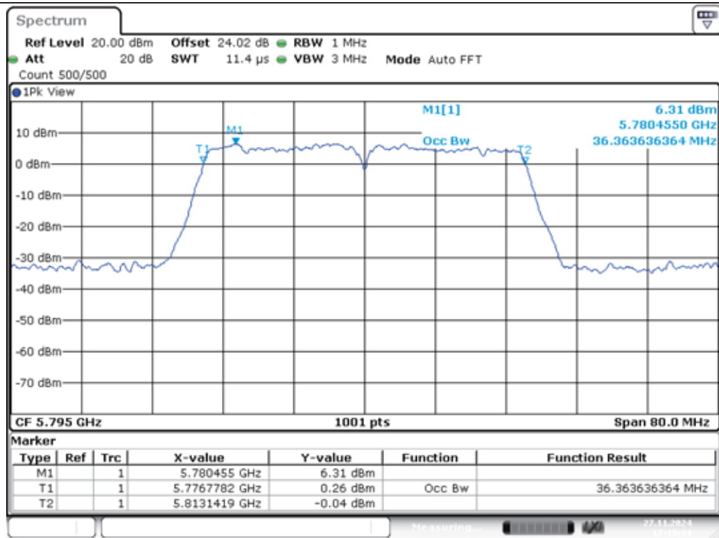
11AC40MIMO-Ant1-5795
