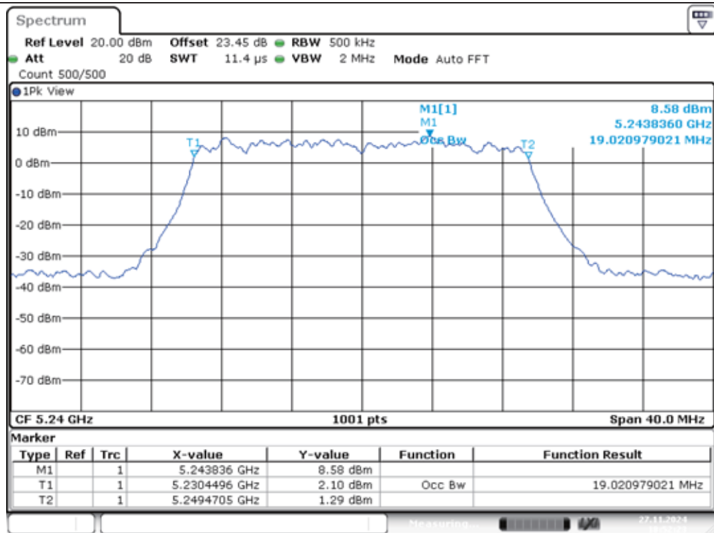
11AX20MIMO-Ant1-5240
