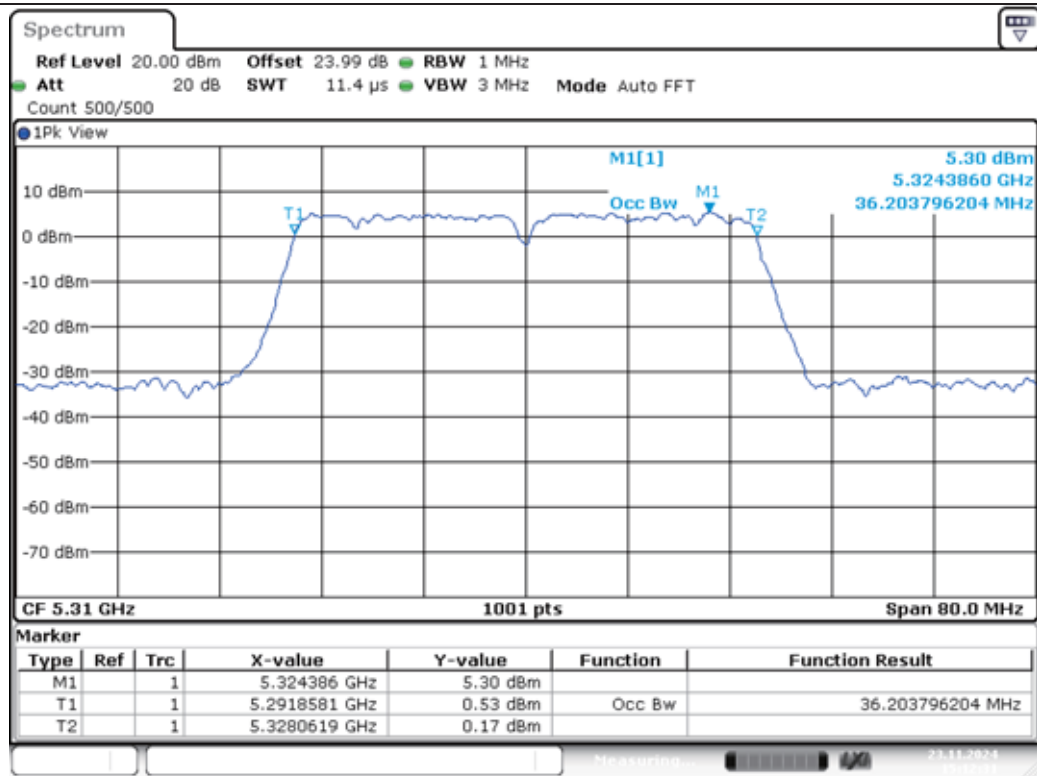
11N40MIMO-Ant1-5310
