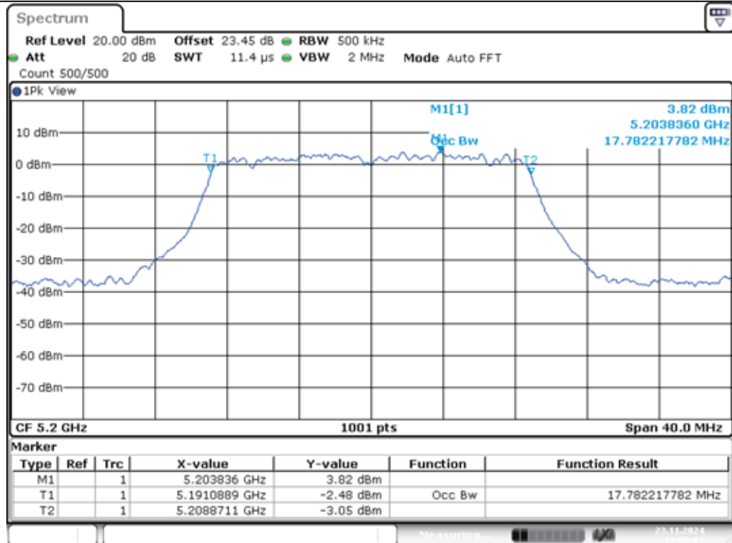
11N20MIMO-Ant1-5200
