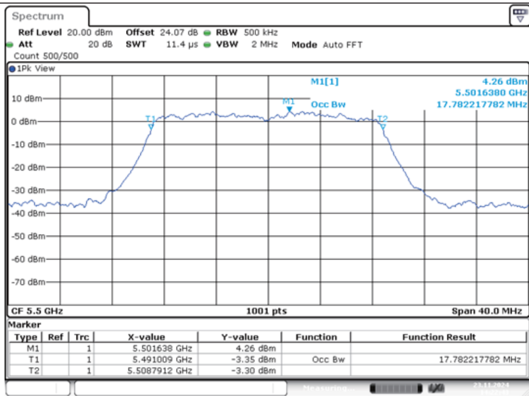
11N20MIMO-Ant1-5500
