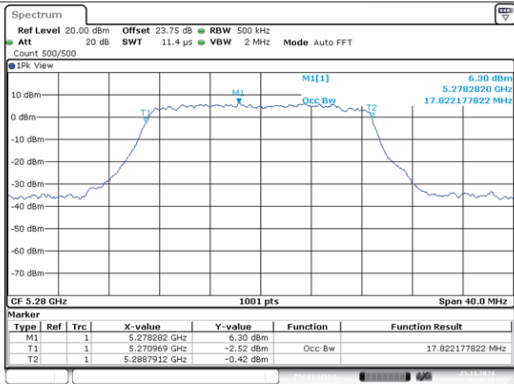
11AC20MIMO-Ant1-5280
