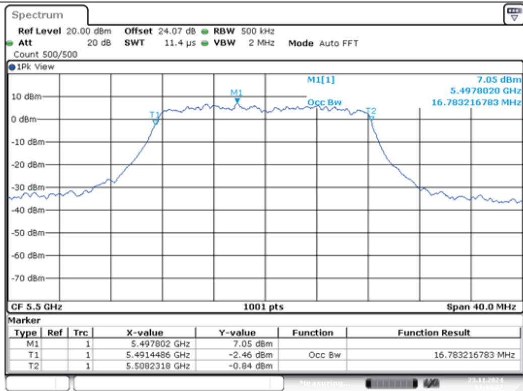
11A-Ant1-5500
