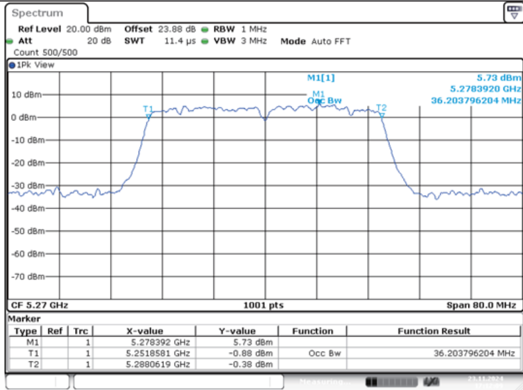
11AC40MIMO-Ant1-5270
