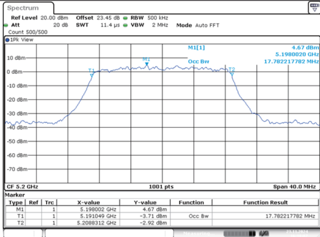
11AC20MIMO-Ant1-5200
