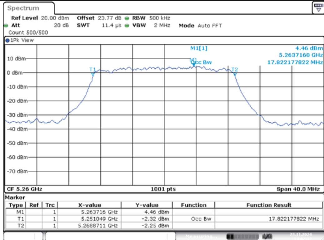
11N20MIMO-Ant1-5260
