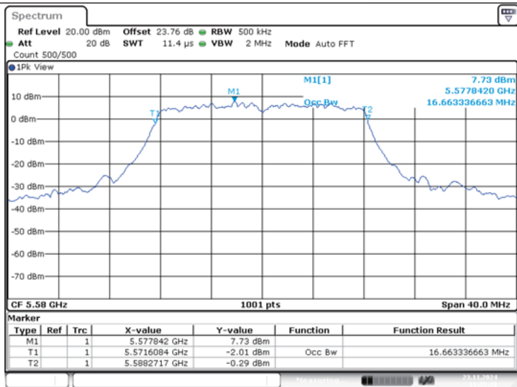
11A-Ant1-5580
