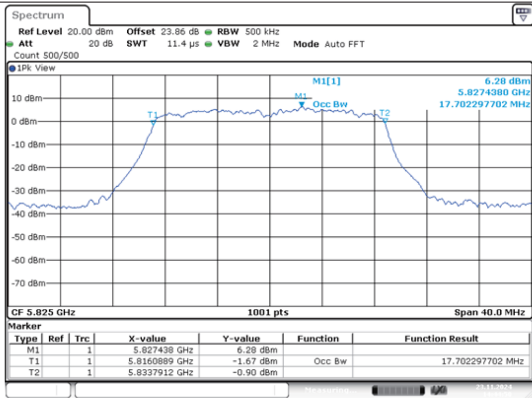
11N20MIMO-Ant1-5825
