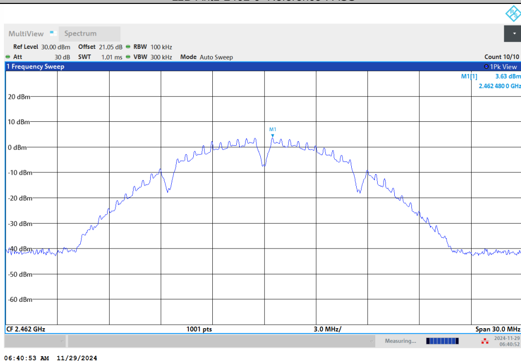
11B-Ant2-2462-0-Reference-PASS
