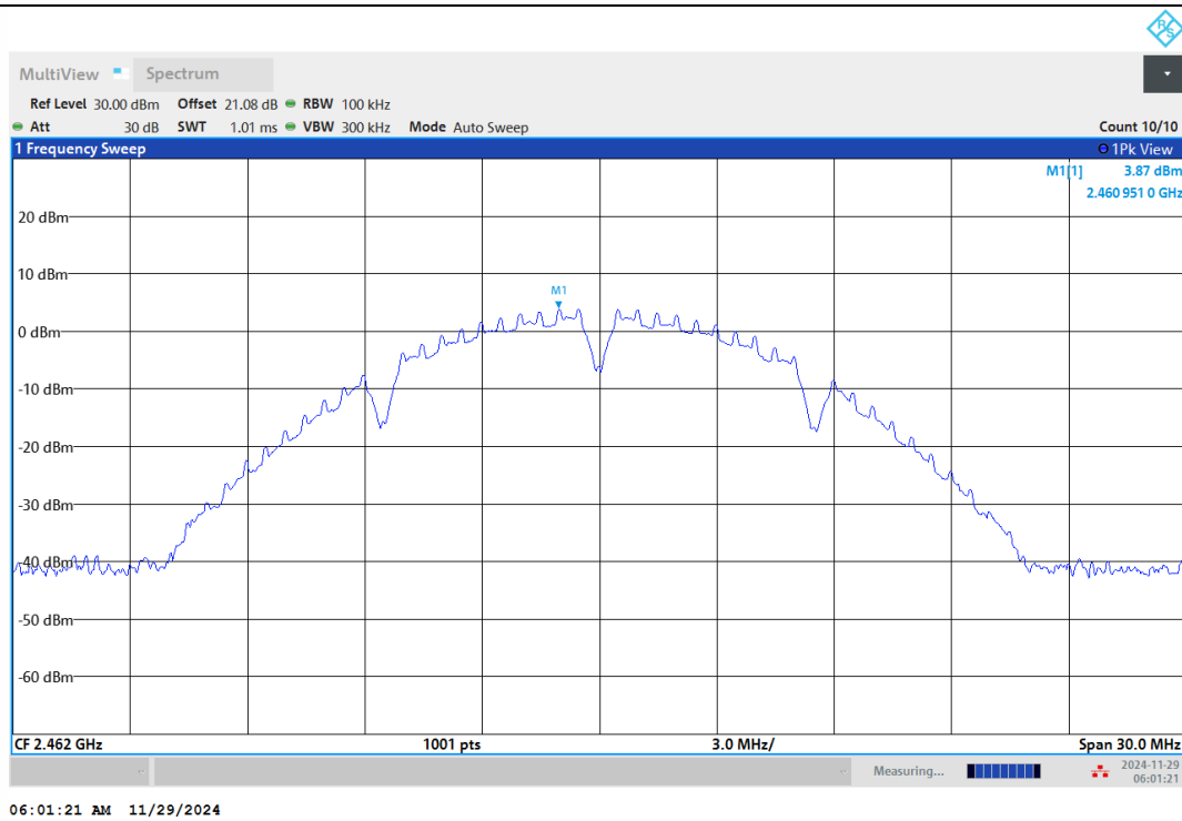
11B-Ant1-2462-0-Reference-PASS
