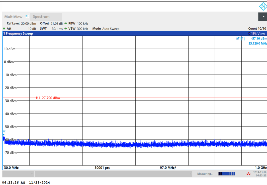
11G-Ant1-2462-30~1000-PASS
