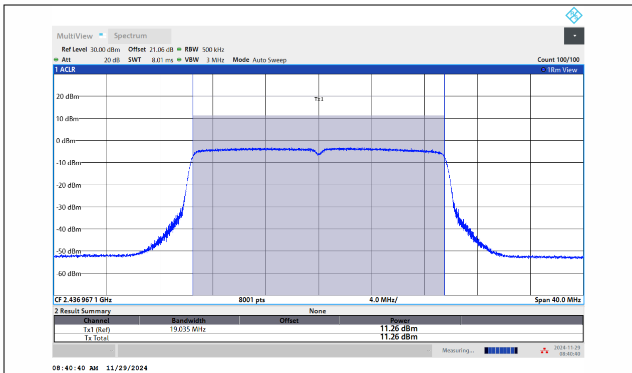
11AX20MIMO-Ant1-2437-PASS
