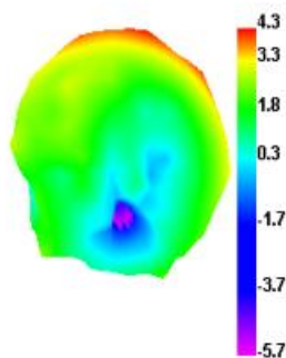
5850.000MHz H
